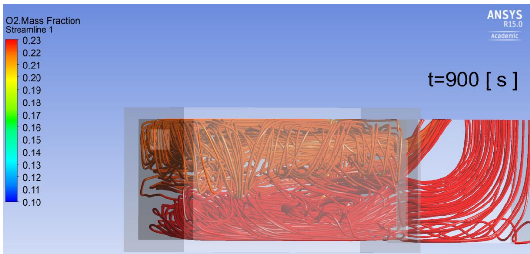
Abbildung 26: Sauerstoffkonzentrationsgefärbte Stromlinien zum Zeitpunkt t=15\text{min}
