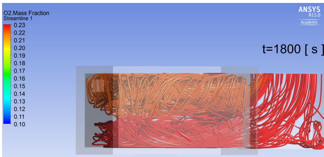
Abbildung 27: Sauerstoffkonzentrationsgefärbte Stromlinien zum Zeitpunkt t=30\text{min} .
