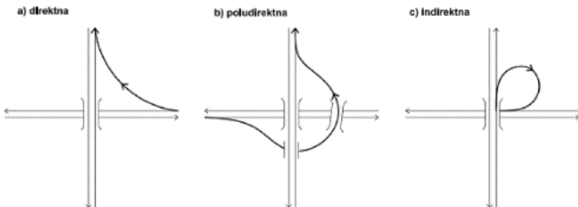
Slika 6. Osnovni oblici spojnih rampi, [1]
