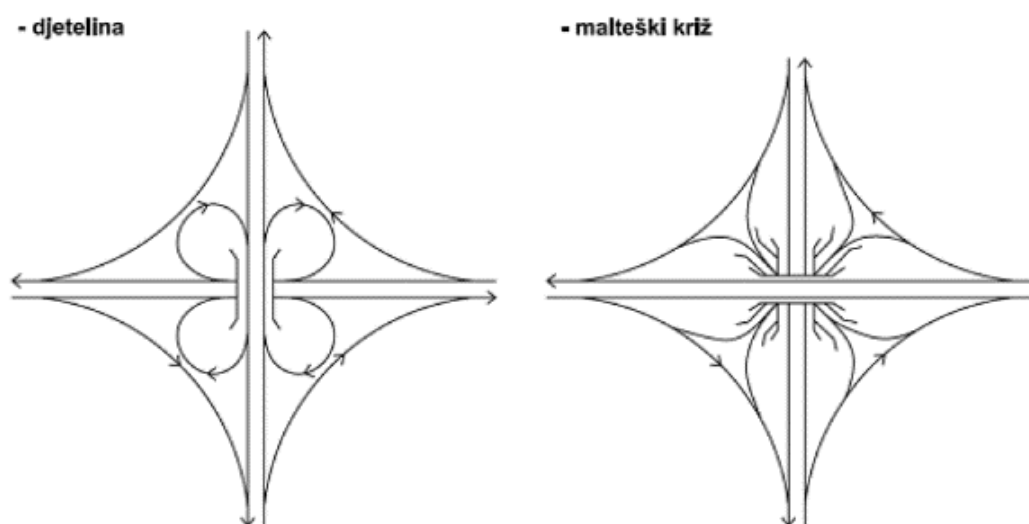
Slika 4. Osnovni modaliteti raskrižja izvan razine s četiri privoza, [1]
