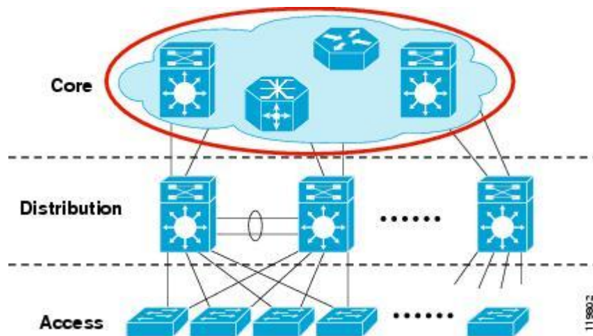
Slika 1. Jezgrena mreža
