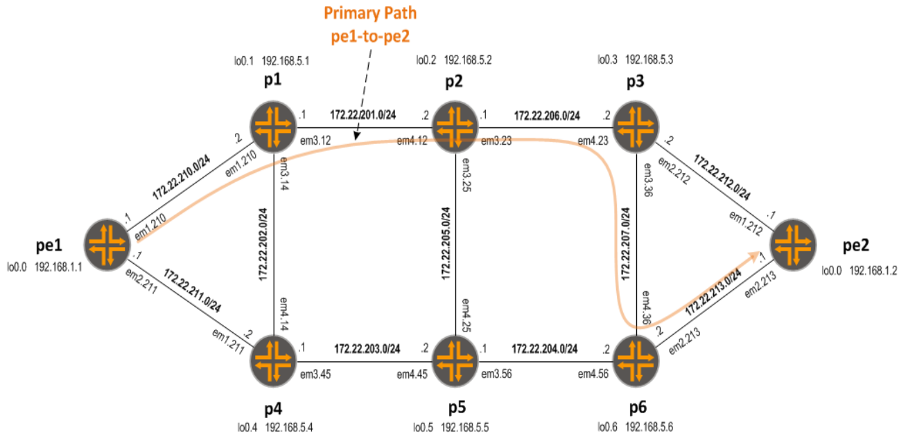
Slika 10. MPLS LSP
