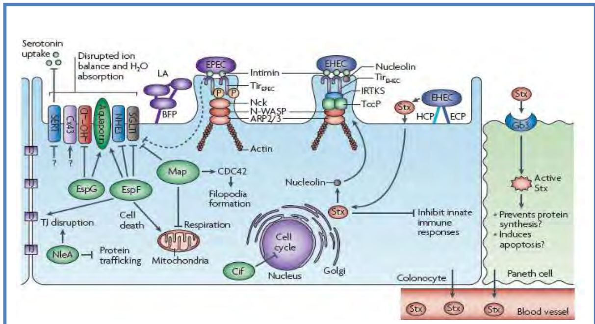
Figure 2.2. Mécanisme de pathogénicité des E. coli entéropathogènes (EPEC) et entérohémorragiques D'après (99)
