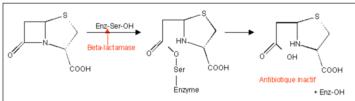
Figure 3.4. Schéma réactionnel de l'ouverture du cycle bêta-lactame
