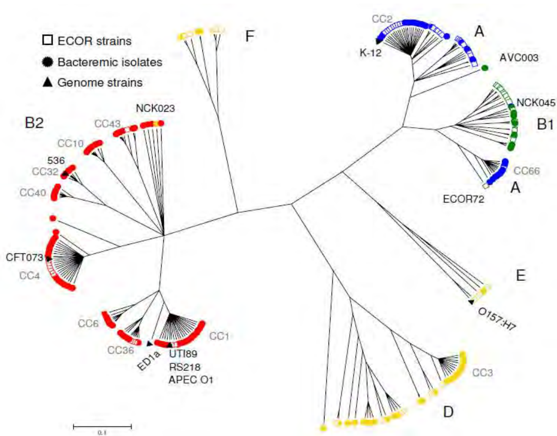
Figure 1.1. Diversité phylogénétique des souches de Escherichia coli
