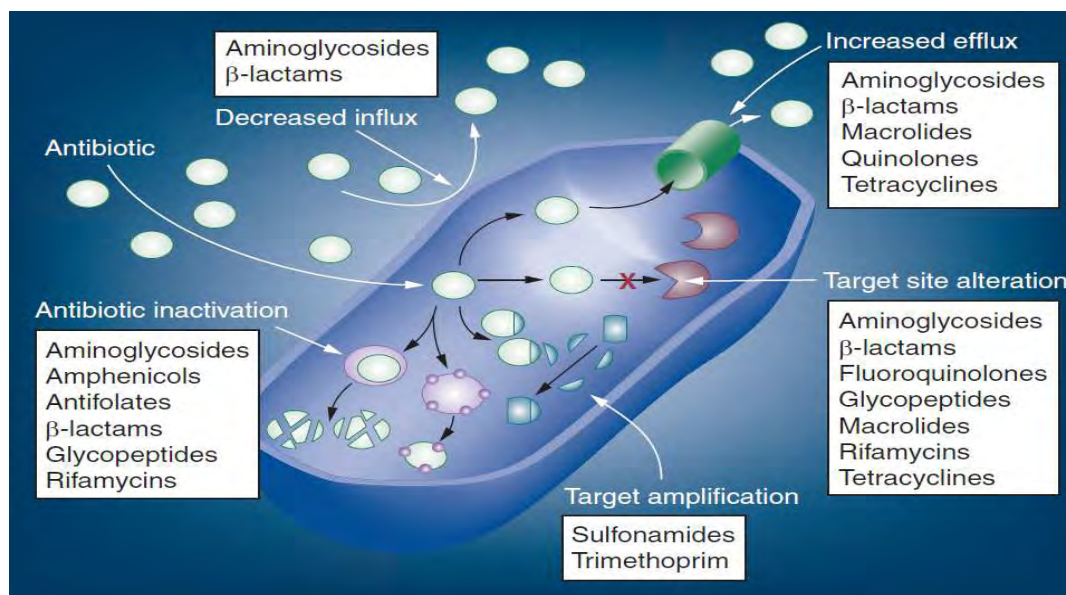
Figure 3.3. Présentation des mécanismes de résistance aux antibiotiques par les bactéries D'après (405)
