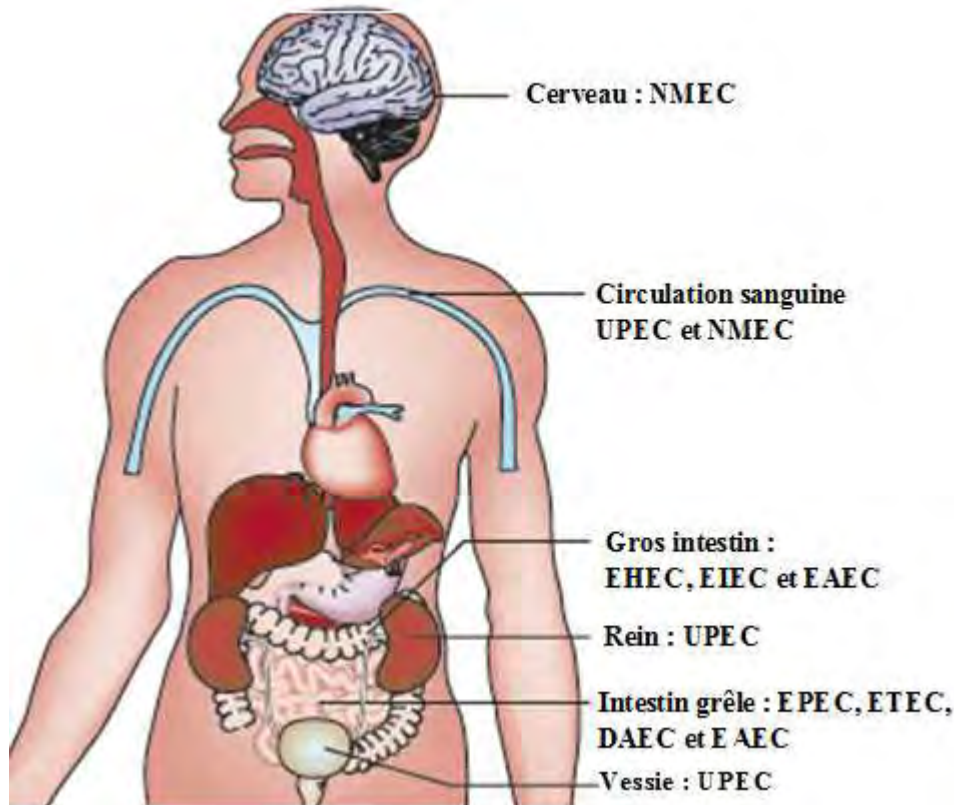
Figure 2.1. Sites de colonisation des Escherichia coli pathogènes
