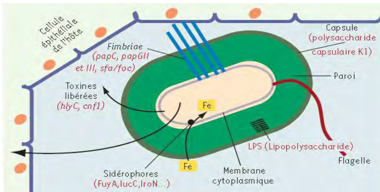
Figure 2.5. Principaux facteurs de virulence impliqués dans le développement des processus infectieux chez les ExPEC D'après (205)
