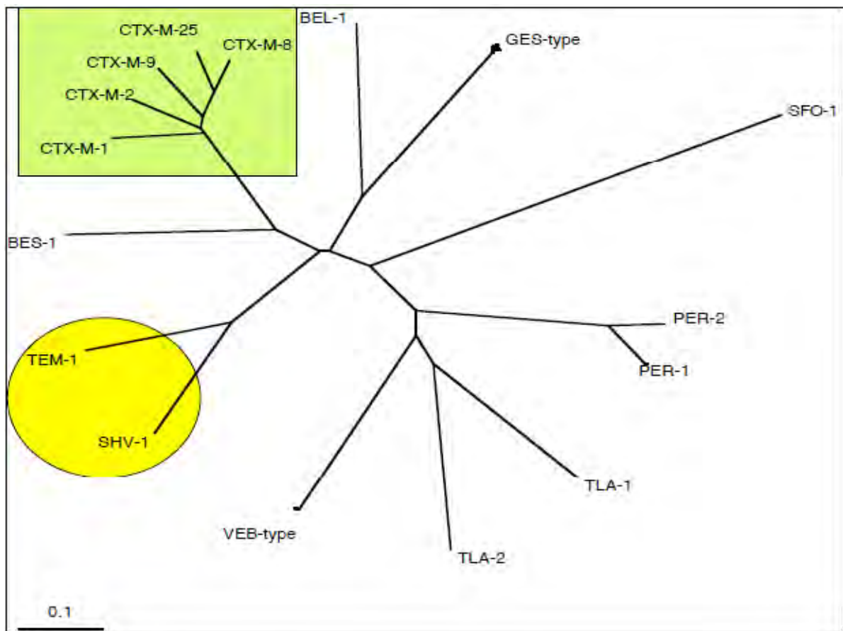
Figure 3.5. Classification phylogénétique des BLSE D'après (147)
