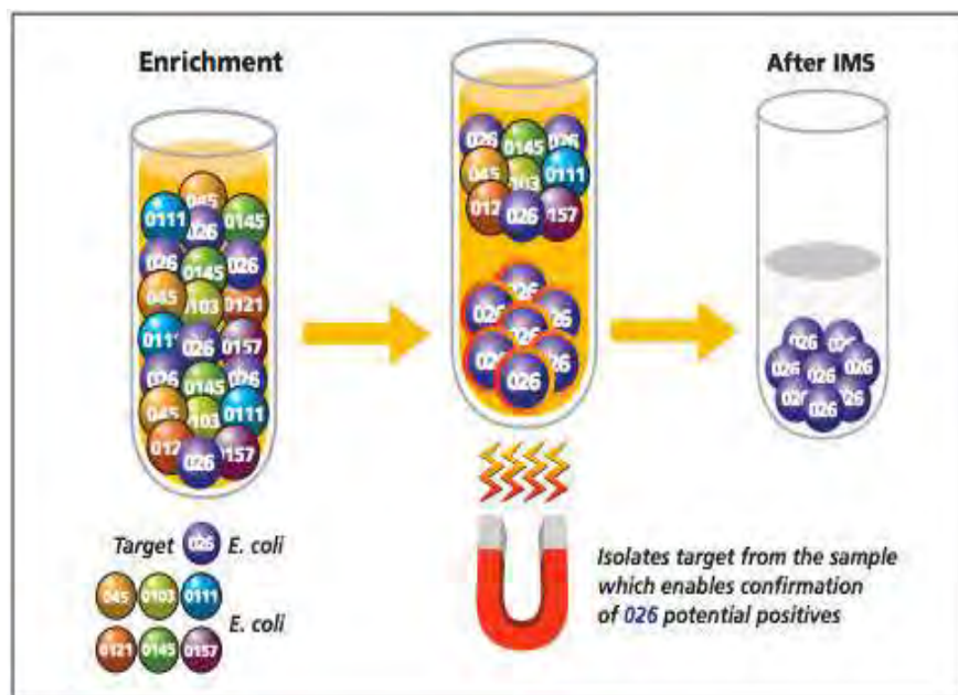
Figure 6.3. Schéma de la réaction d'immuno séparation magnétique
