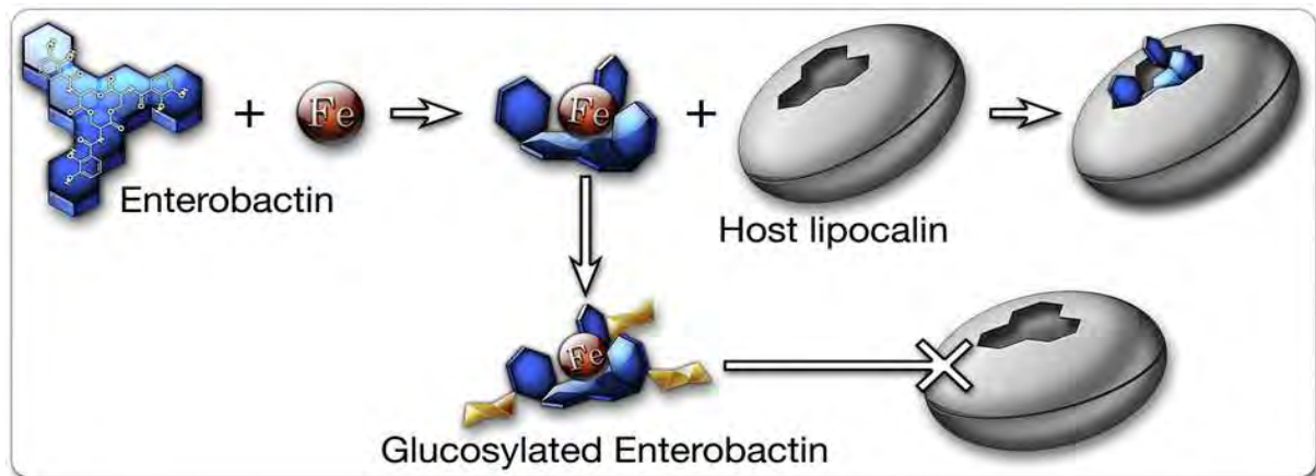
Figure 2.7. Mécanisme de compétition pour le fer entre l'entérobactine, la lipocaline 2 et la salmochéline. Lorsque l'entérobactine est liée au fer, elle est séquestrée par la lipocaline 2 et n'est alors plus disponible pour les bactéries qui l'ont secrétée. En revanche, la forme glycosylée de l'entérobactine, la salmochéline, ne peut être captée par la lipocaline 2 et reste donc un sidérophore efficace pour les bactéries. Adaptée de (472)
