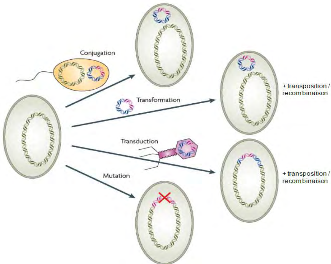
Figure 3.1. Les trois modes de transmission du matériel génétique : la conjugaison, la transformation et la transduction chez les bactéries.
