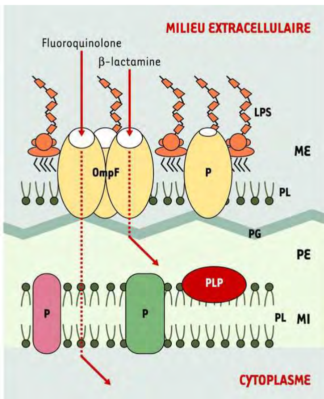
Figure 3.2. Enveloppe de Escherichia coli
