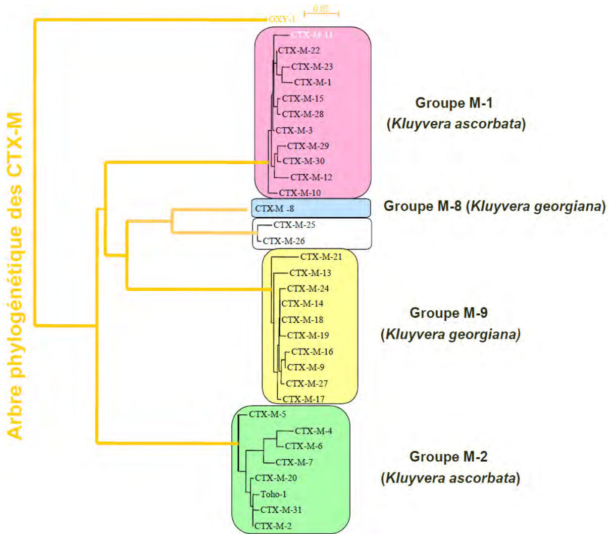
Figure 3.6. Schéma de l'arbre phylogénétique des CTX-M : Origine des gènes codant le groupe CTX-M D'après (147)
