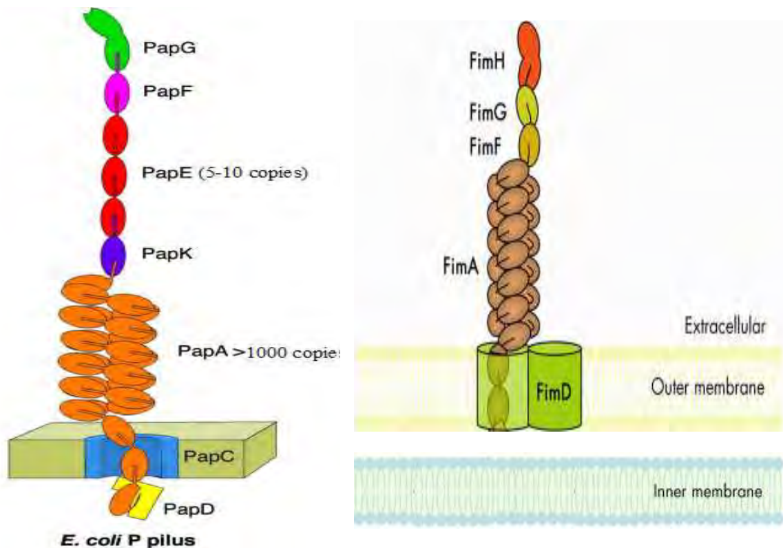
Figure 2.6. Structure des fimbriae de type 1 et des fimbriae de type P
