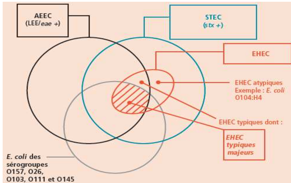
Figure 2.3. Représentation schématique des souches AEEC, EHEC et STEC
