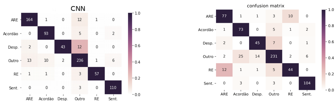
(a) Matriz de confusão CNN. Fonte: (SILVA et al., 2018, p. 3)
