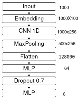
(a) Modelo baseado em CNN (SILVA et al., 2018).
