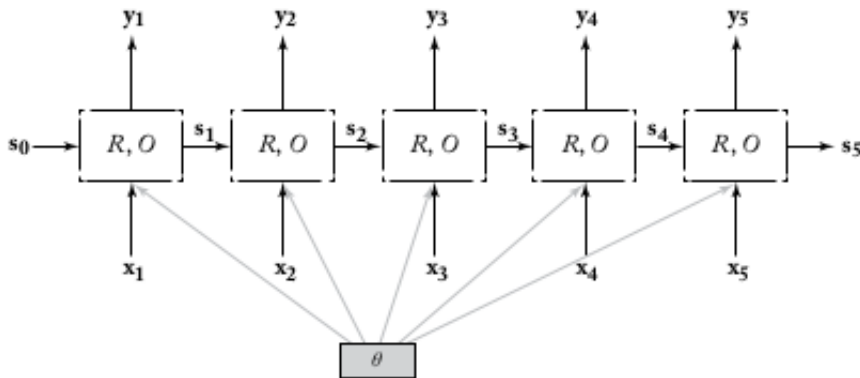
Figura 11 – Arquitetura recursiva da RNN. Fonte: Goldberg (2017, Página 166)
