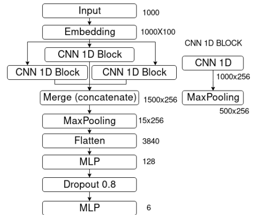
(b) Modelo baseado em CNN (KIM, 2014).
