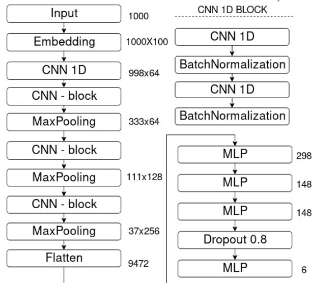
(c) Modelo baseado em CNN (CONNEAU et al., 2017).
