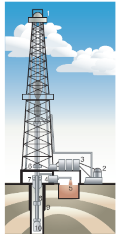
Figura 1: Esquema de uma torre de perfuração: 1 - bloco de coroamento, 2 - bomba de lama, 3 - motores, 4 - peneira, 5 - tanque de lama, 6 - mesa rotativa, 7 - válvula de segurança, 8 - tubo de perfuração, 9 - tubo de revestimento e 10 - broca de perfuração.
