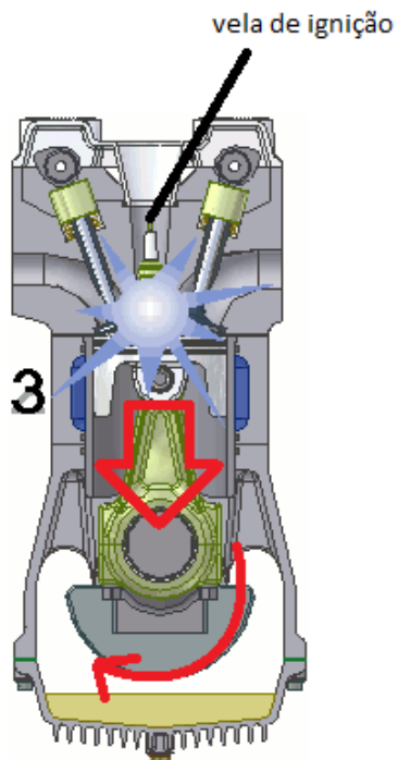
Figura 3 – Motor de 4 tempos - 3° Tempo
