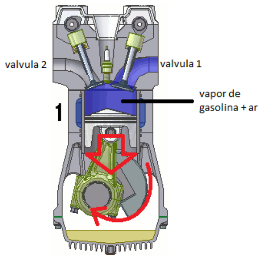
Figura 1 – Motor de 4 tempos - 1° Tempo
