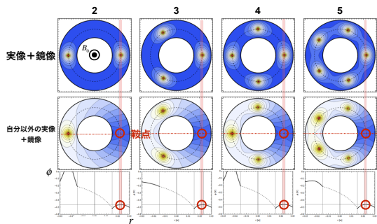
図4. 二重同軸境界における不安定平衡解
