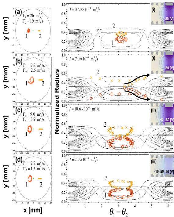
図3. 二本の電子渦糸の実空間(左)と位相空間(右)における軌道。右図の等高線はオイラー流体の理論から計算したハミルトニアン一定の軌道を表す。
