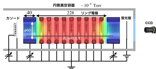
図 2. 電子プラズマ閉じ込め装置。左側のカソードから入射した電子群は、赤で示した領域に閉じ込められる。右側の蛍光面の輝度分布を CCD カメラで撮影する。
