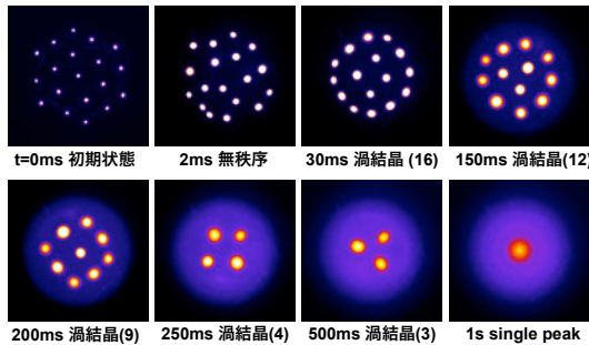
図 1. 非中性プラズマで見られる渦結晶
