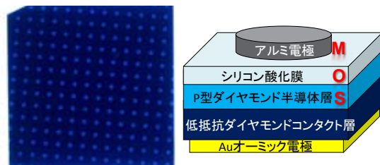
図 現在開発中のダイヤモンドMOSダイオードの外観(左)とその模式図(右)
