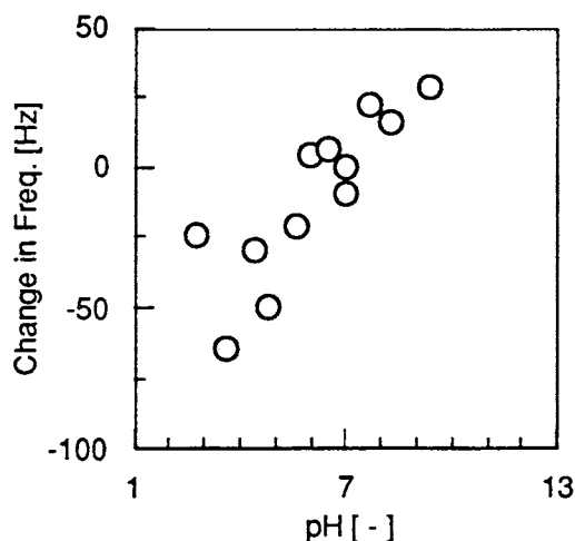
図9 溶液pHと振動数変化の関係
