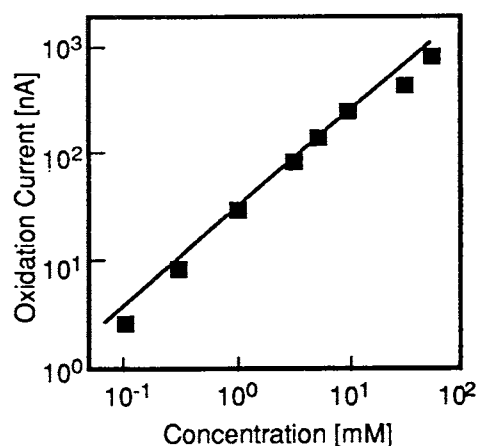
図12 フェロセンを電子メディエータとして用いた場合のグルコース濃度と酸化電流の直線関係
