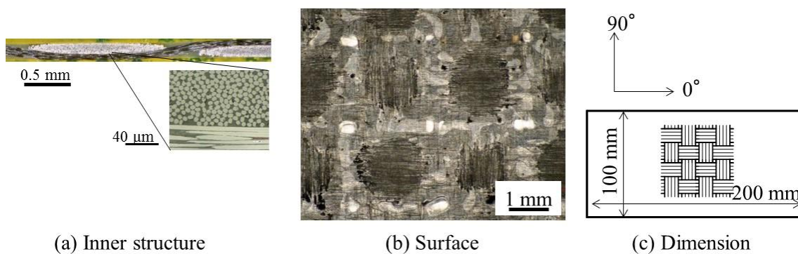
Fig. 2 CFRTP sheet
