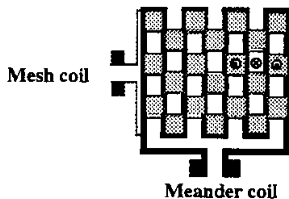
(d) Detection of variance flux using a mesh coil
