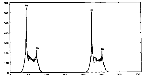
図7 フィードバックで s_1 成分をキャンセルしたヒストグラム
