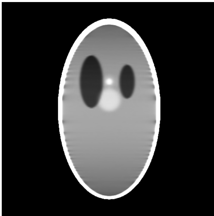
Abbildung 3.2.5.b): Rekonstruktion der Ebene y = 0.102 , Radius der Abtastkurve: r = 12 .
