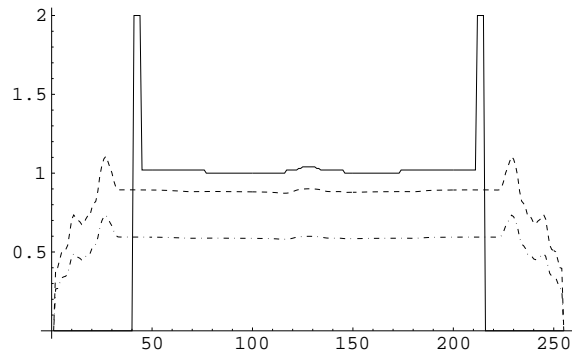
Abbildung 2.3.4: Querschnitt durch das Shepp-Logan-Phantom: durchgezogene Linie: Original-Werte, gestrichelt: Rekonstruktion mit Korrekturterm, gepunktet: Rekonstruktion ohne Korrekturterm.
