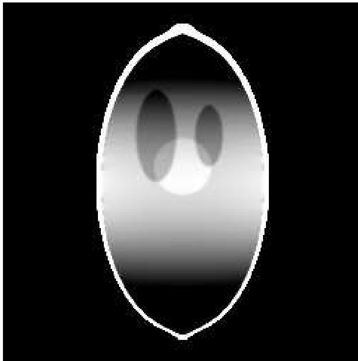
Abbildung 3.2.5.a): Rekonstruktion der Ebene y = 0 .
