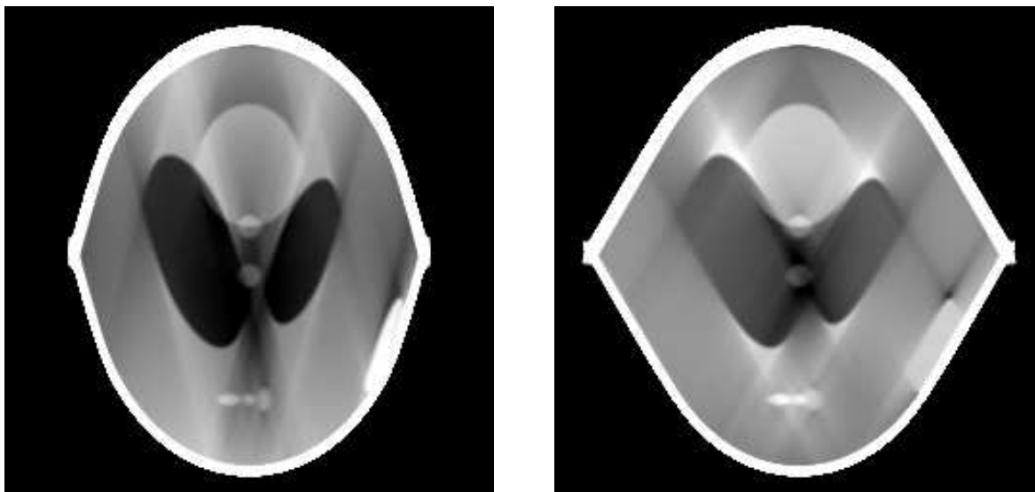
Abbildung 2.3.2: Rekonstruktion mit 255 \times 255 Bildpunkten für \Phi = \pi/12 (links) bzw. \Phi = \pi/6 (rechts).
