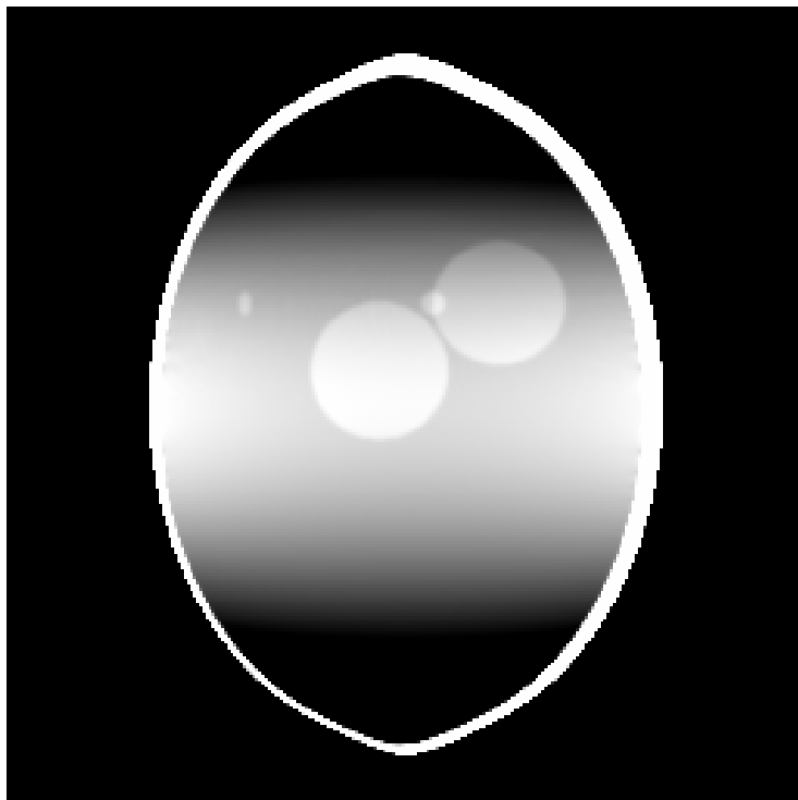
Abbildung 3.2.4: Rekonstruktion der Ebene x = 0 .
