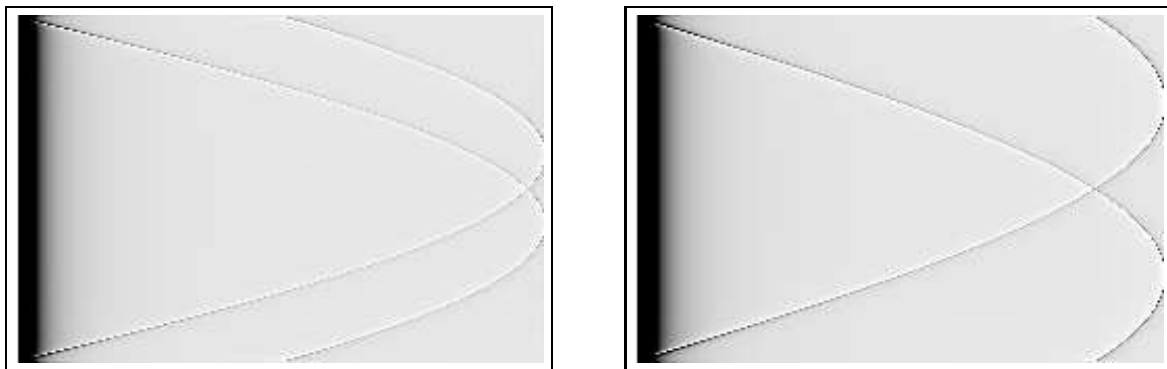
Abbildung 2.3.1: Density-Plot der Rekonstruktionskerne für \gamma = 0.0031 und \Phi = \pi/12 (links) bzw. \Phi = \pi/6 (rechts): die horizontale Richtung ist die s -Richtung im Intervall [0, 1] , die vertikale Richtung die \varphi -Richtung im Intervall [\Phi, \pi - \Phi] .
