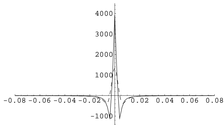
Abbildung 2.1.2: Rekonstruktionskern für \gamma = 0.0031 (gestrichelt) und \gamma = 0.0018 .
