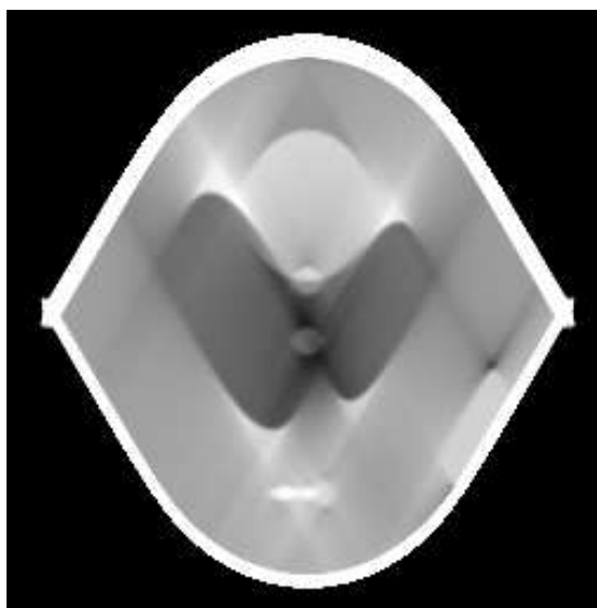
Abbildung 2.3.3: Rekonstruktion für \Phi = \pi/6 ohne Verwendung des Korrekturterms.
