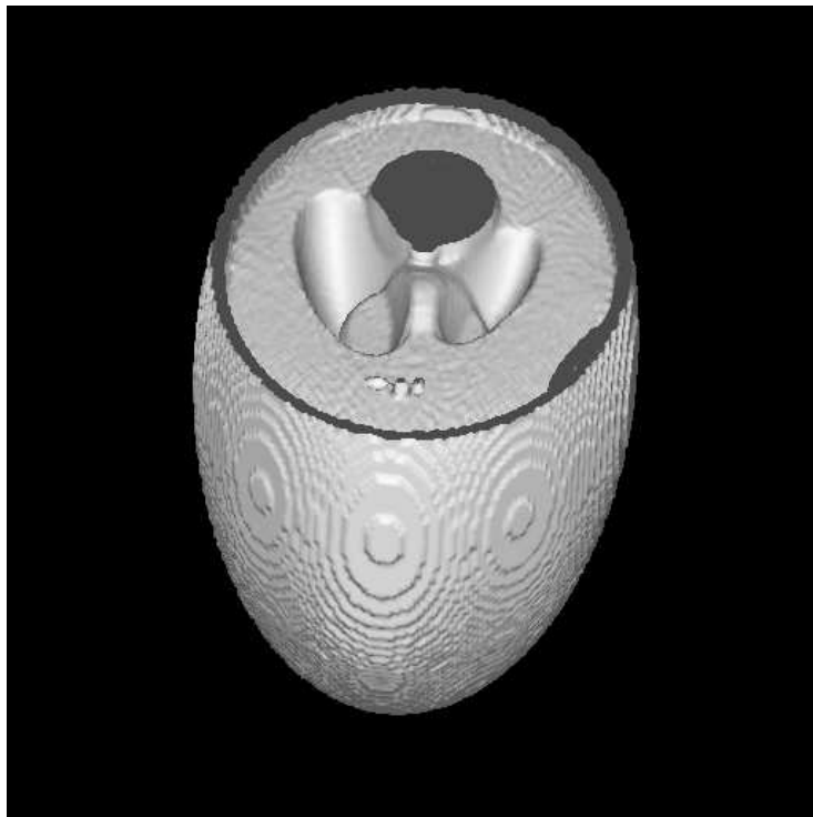
Abbildung 3.2.3: Dreidimensionale Darstellung des originalen Shepp-Phantoms.
