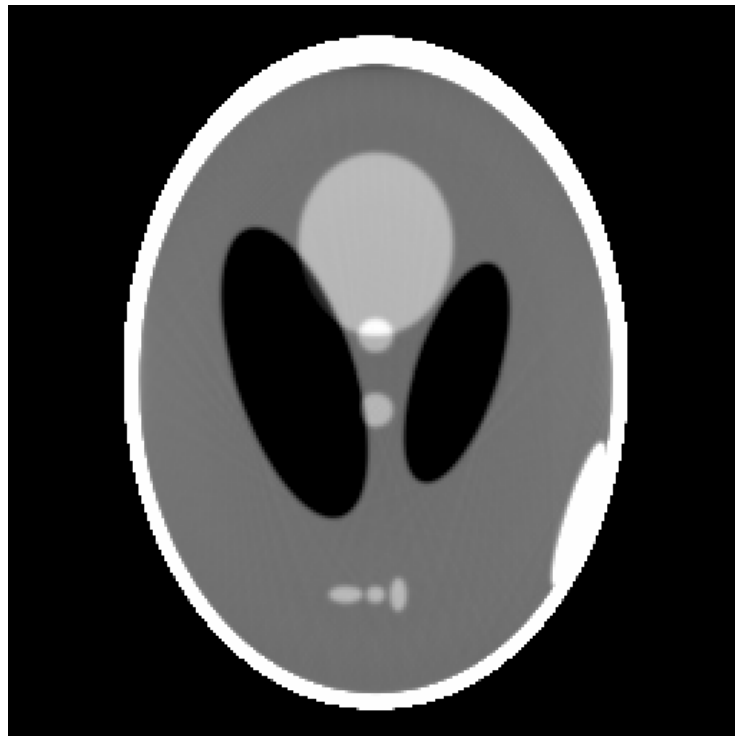
Abbildung 2.1.4: Rekonstruktion aus von 200 Richtungen mit 255 Strahlen pro Richtung gemessenen Daten.
