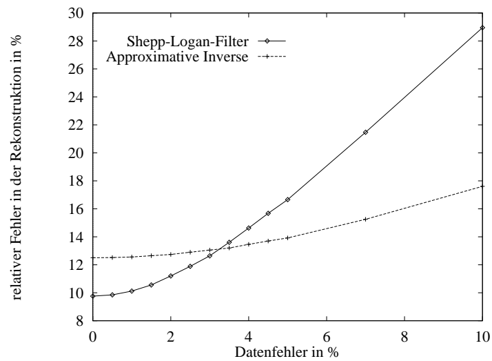
Abbildung 2.1.9: Vergleich der Rekonstruktionen mit verrauschten Daten.
