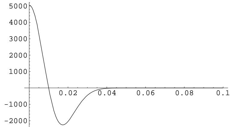
Abbildung 3.2.1: Rekonstruktionskern für die 3D-Radon-Transformation, \gamma = 0.01 .
