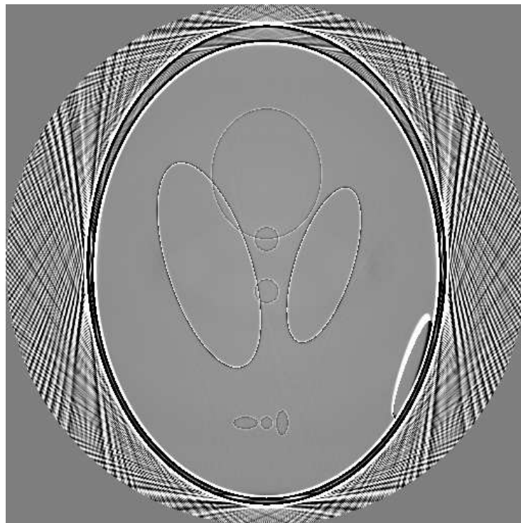
Abbildung 2.1.10: Differenz des Originalbildes (Abbildung 2.1.3) und des rekonstruierten Bildes (Abbildung 2.1.5).
