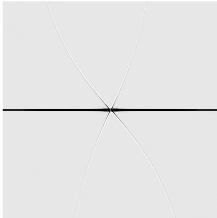
Abbildung 3.2.2.a): Kern \tilde{k}(0; a_0, \theta) .
