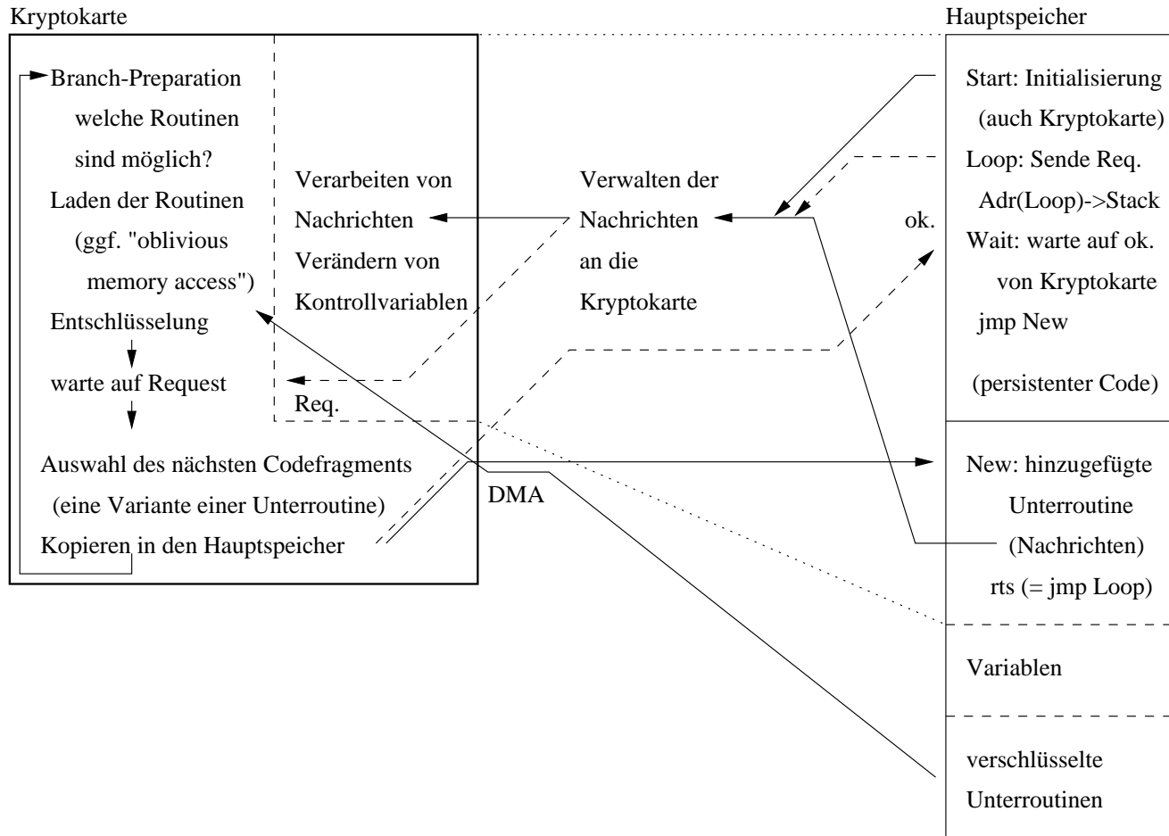
Abbildung 1: Abarbeitung eines geschützten Programms
