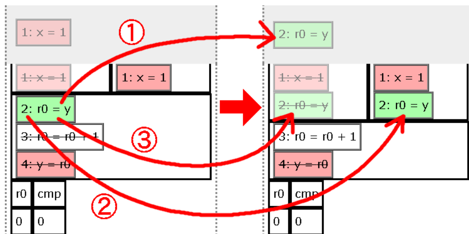
図 5.10: OoO 実行のアニメーション (機械命令のフェッチ・デコード): ①実行履歴への配置, ②リザーベーション・ステーションへのコピー, ③リオーダー・バッファへのコピー
