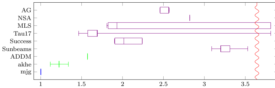
Fig. 8: VeRoLog_late_r1000d25_3
