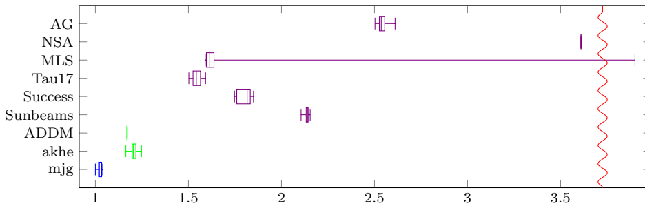
Fig. 9: VeRoLog_late_r1000d25_4
