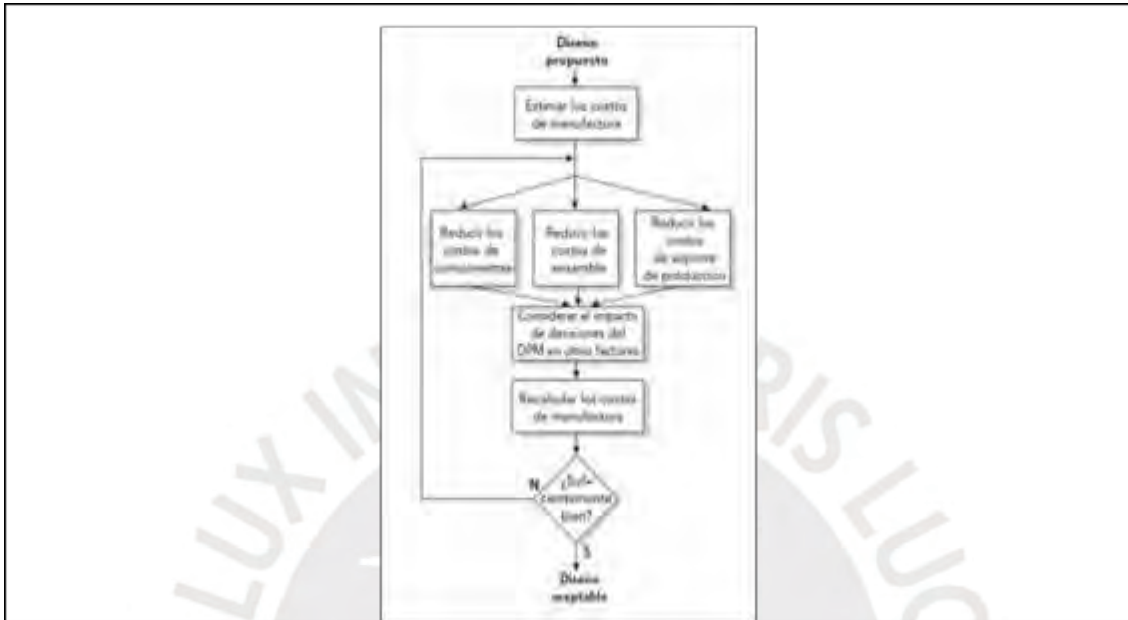
Figura XXI: Etapas del proceso de diseño de manufactura
