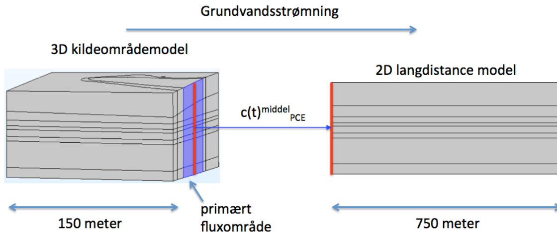
Figur 3 – Konceptuel fremstilling af 3D- og 2D-modeller med kobling mellem de to markeret som rød linie. Bemærk: Størrelsesforhold harmonerer ikke.
