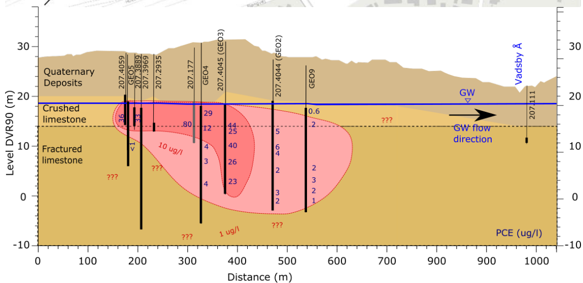
Figur 34 - Målte PCE koncentrationer i fanen fra Akacievej 2 i vinteren 2014, mens afværgen er i drift. Den horisontale udbredelse er i den knuste kalk (overgangen til sprækket kalk). Den vertikale udbredelse er langs en vurderet central strømningslinje. Koncentrationsdata stammer fra Broholm et al. (2016).
