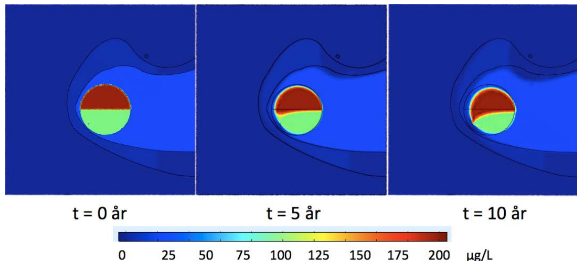
Figur 15 – Simuleret PCE-koncentration set ovenfra cirka midt i den knuste kalk efter 0, 5 og 10 år. Med afværgelanlæg aktiveret (S1).
