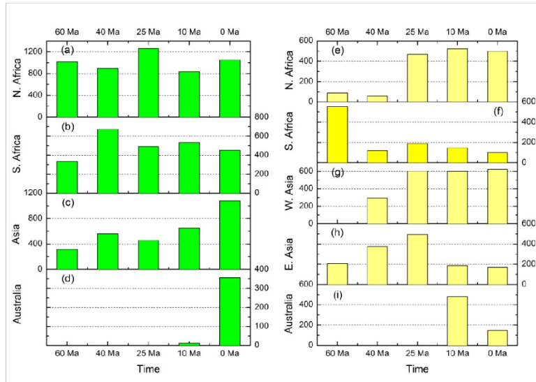
图 3 新生代 5 个时期 4 个季风区面积变化 (左列), (a) 北非季风区, (b) 南非季风区, (c) 亚洲季风区, (d) 澳洲季风区; 以及 5 个干旱区面积变化 (右列), (e) 北非干旱区, (f) 南非干旱区, (g) 西亚干旱区 (亚洲 70°E 以西), (h) 东亚干旱区 (亚洲 70°E 以东), (i) 澳洲干旱区。面积单位为 10^4 \text{ km}^2 。
