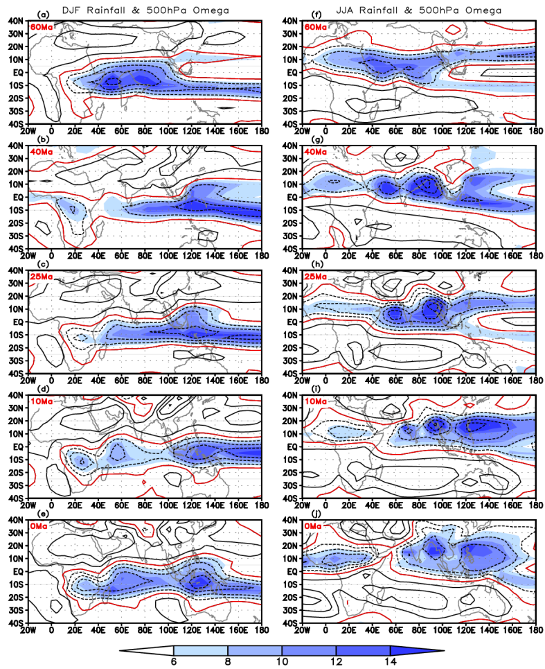
图 4 60Ma、40Ma、25Ma、10Ma 和 0Ma 北半球冬季 (DJF) 平均 (左列) 和夏季 (JJA) 平均 (右列) 降水率 (阴影, mm/d) 和 500 hPa 垂直速度 (等值线, 间隔为 0.01 Pa/s, 红线为零线, 负值指示上升运动) 分布
