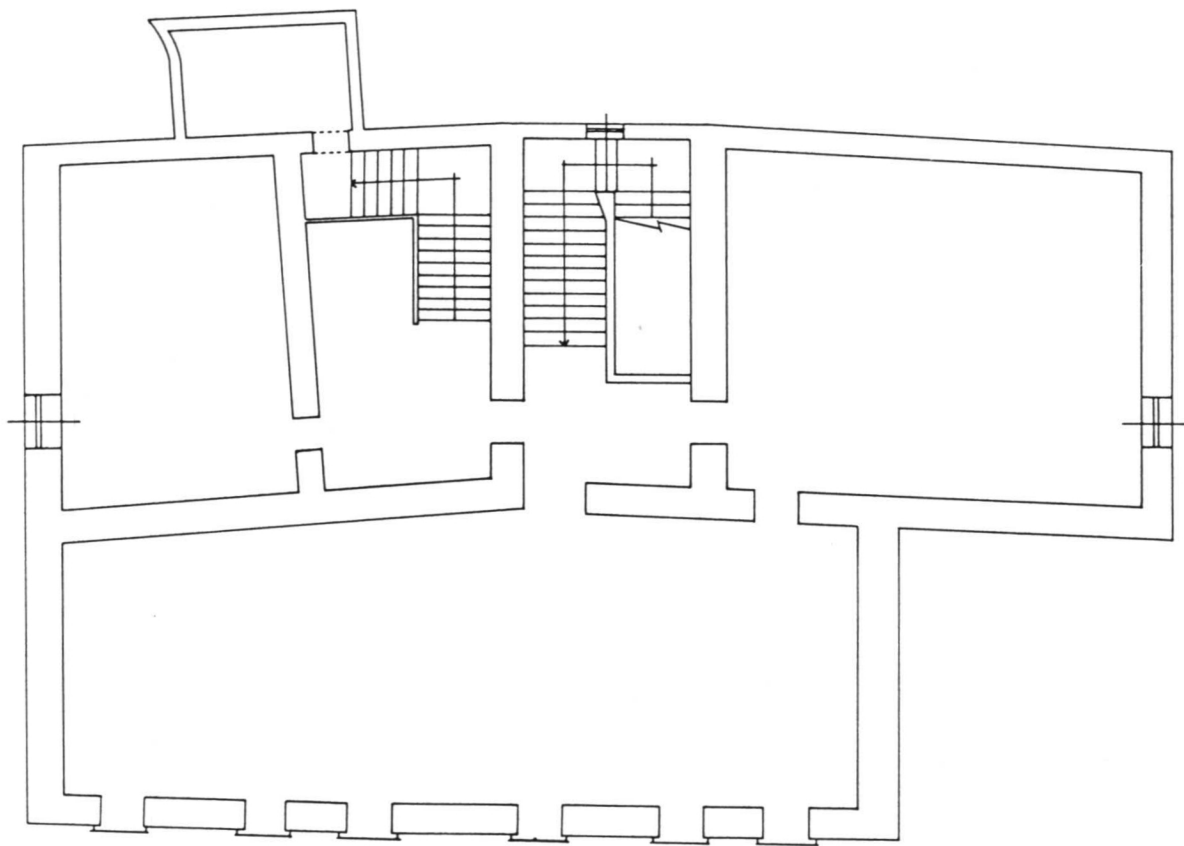
Lámina 3. Alhóndiga de Plasencia. Planta principal.
