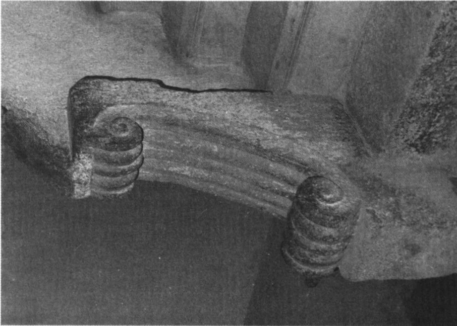
6. Ménsula-machón de la escalera.
