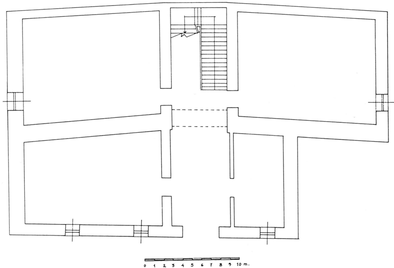
Lámina 2. Alhondiga de Plasencia. Planta baja.
