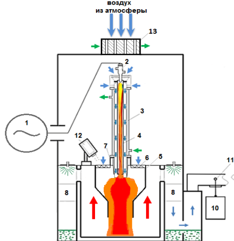
Рис. 1. Схема плазменного модуля на базе ВЧФ-плазмотрона.
