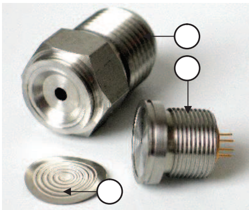
Slika 5 - Elementi transdjusera pritiska: 1) procesni priključak, 2) membrana, 3) centralna sekcija sa izvodnicama
