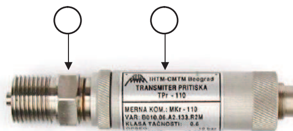
Slika 2 - Transmitter pritiska TPr-110: 1) merna komora, 2) kutija elektronike
