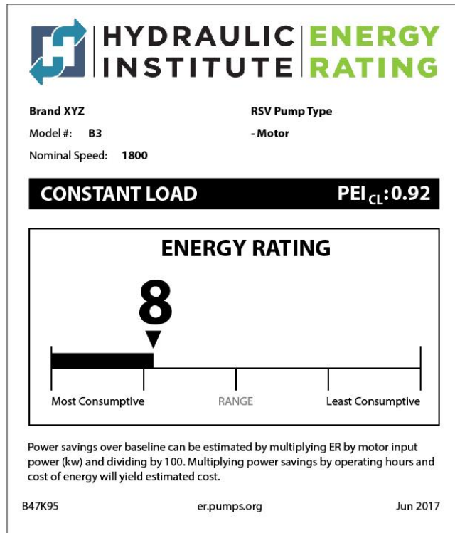
Figure 10. HI ER Label
