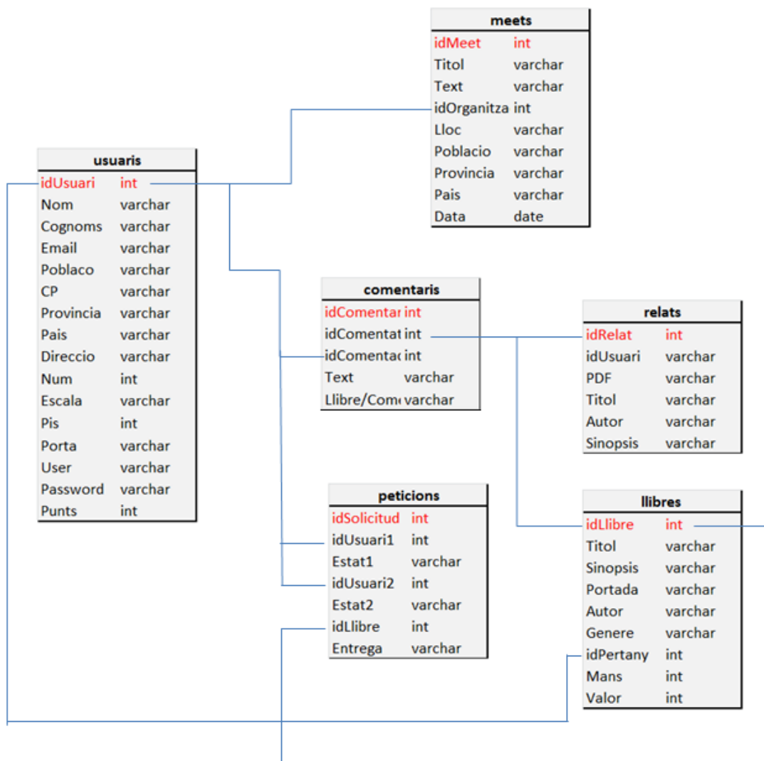
Figura 6 - Diagrama d'entitat-relació representatiu de la base de dades
