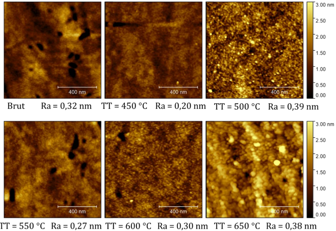
Figure 3-5 : Micrographies AFM de la couche mince brute et des couches minces d'épaisseurs 300 nm recuites sous vide primaire.
