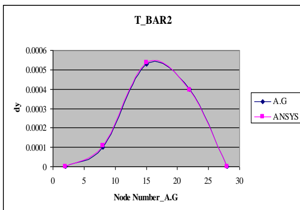
شکل ۱۰: مقایسه جابجایی به دست آمده در گره های مشخص در راستای y
