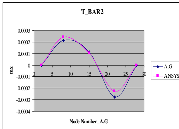
شکل ۹: مقایسه ممان پیچشی به دست آمده در گره های مشخص در راستای x
