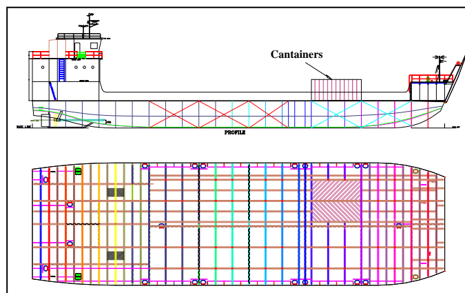
شکل ۸. جانمایی کلی و نما از عرشه شناور حامل کانتینر
