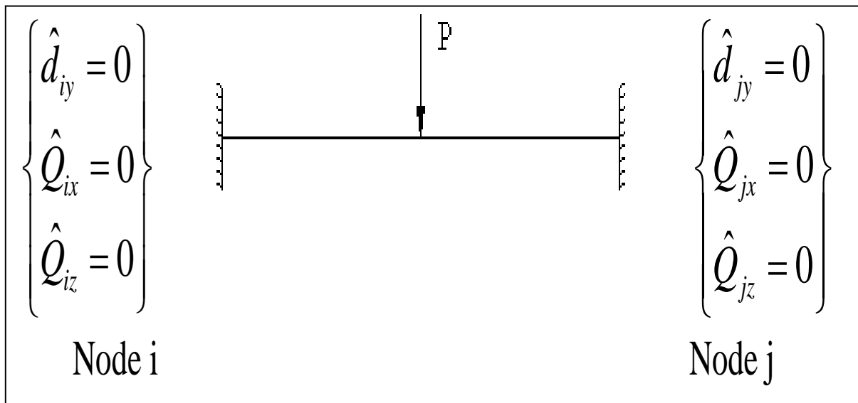
شکل ۴. شرایط مرزی ثابت یا گیردار
