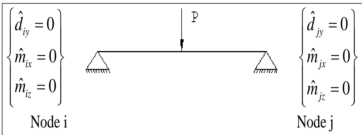
شکل ۵. شرایط مرزی ساده
