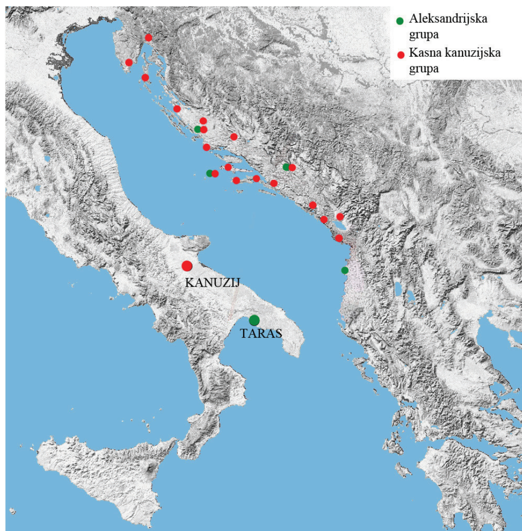
Karta 2: Distribucija Aleksandrijske i Kasne kanuzijske grupe
