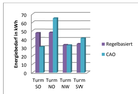
Abbildung 5 Vergleich mit dem regelbasierten Regler - Energiebedarf
