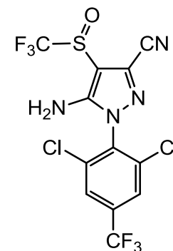
Fipronil (18)
