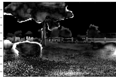
(j) error 2
