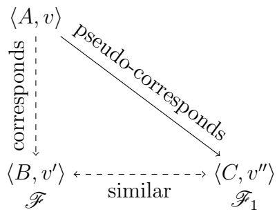
Figure 2: Lemma 5
