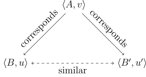
Figure 3: Lemma 8
