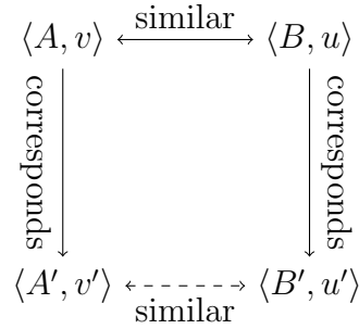
Figure 4: Lemma 10
