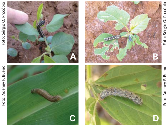
Figura 2. Lagartas do gênero Spodoptera de importância econômica no Brasil. (A) Spodoptera cosmioides , (B) Spodoptera eridania , (C) Spodoptera frugiperda , (D) Spodoptera albula .
