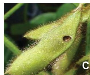
Figura 1. Redução do estande inicial (A), desfolha (B) e ataque à vagem (C) de plantas de soja por Spodoptera spp.
