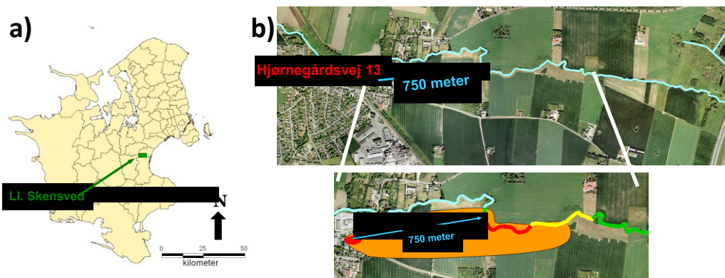
Figur 13: a) Oversigtskort over Sjælland, der viser beliggenheden af Ll. Skensved i Danmark. b) Oversigtskort over Hjørnegårdsvej 13 samt den forurenede TCE fane, der spredte sig med den østliggående grundvandstrømning hen til det nærliggende vandløb, Skensved Å. Den rødt markerede del af vandløbet viser området, hvor det indsvivende grundvand havde de højeste TCE koncentrationer (McKnight et al. 2010).
