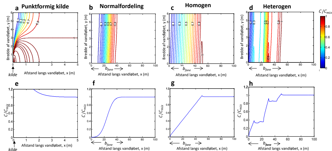
Figur 4: Den normaliserede koncentration i overfladevandet langs vandløbet er vist for de fire forskellige fordelingsfunktioner (punktformig kilde, Guassian, homogen og heterogen) for en forureningsfane ( b_{fane}=50 m og J=4 kg/år) i et typisk mellemstort dansk vandløb ( Q_{vandløb} = 100 L/s, b_{vandløb}= 6 m og d_{vandløb}= 1,5 m). Indsivningen i vandløbet sker fra brinken (x-aksen), og det er antaget, at koncentrationen er ligeligt fordelt over dybden. Bemærk at for en punktformig kilde er der kun vist de første 5 m i vandløbet. Koncentrationerne er normaliseret med den fuldstændigt opblandede koncentration.
