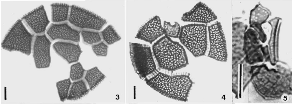
Figs. 3-5.— Peridinium gatunense del Lago Kinneret (previamente denominado P. cinctum f. westii ). 3: placas de la epiteca; 4: placas de la hipoteca + Sp.; 5: placas sulcales. Microscopio óptico; escala 10 micras.
