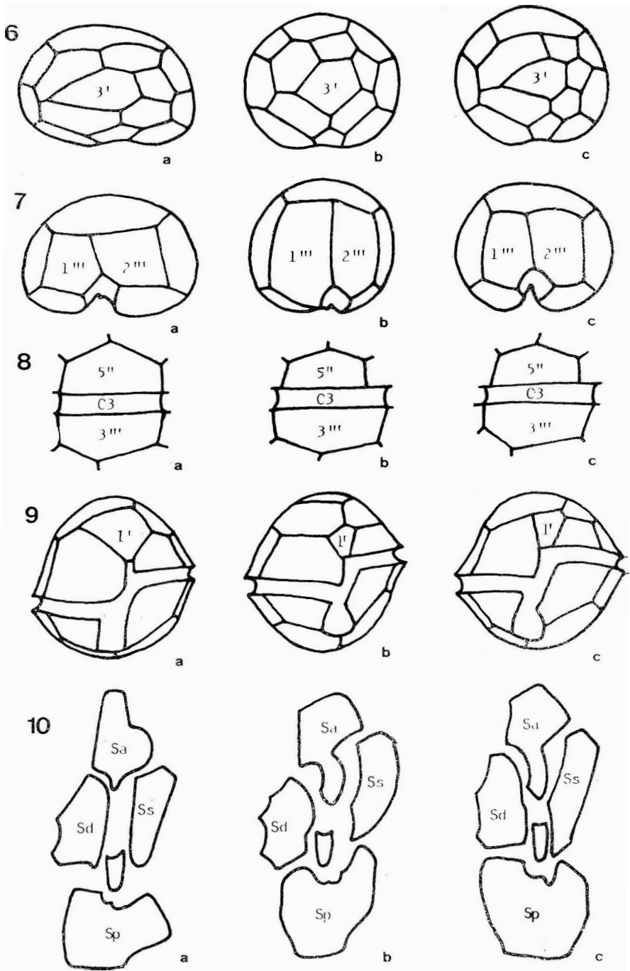
Figs. 6-10. — Esquemas comparativos entre (a) Peridinium cinctum (Tierra del Fuego, Argentina), (b) P. gatunense (Córdoba, Argentina) y (c) P. gatunense (Lago Kinneret, Israel). 6: epiteca; 7: hipoteca; 8: detalle de las placas dorsales; 9: vista ventral; 10: placas sulcales.
