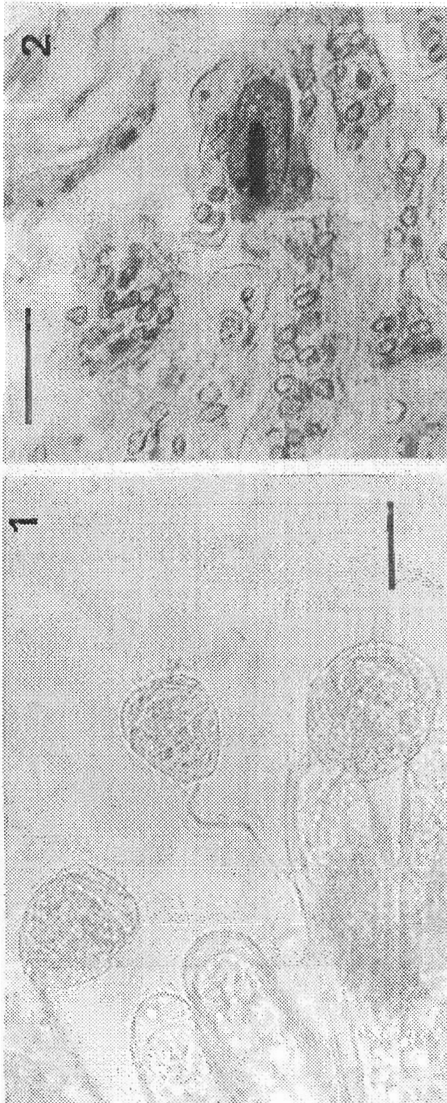
Fig.1: Microfotografía de Vorticella sp. sobre los filamentos branquiales de A. longinaria . Escala = 20 \mu m.
