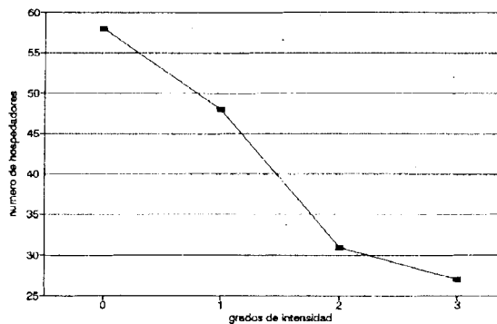
Fig. 7: Distribución de apostomados en las branquias de A. longinaris de acuerdo a los grados de intensidad. 0=no parasitado, 1=poco parasitado; 2=moderadamente parasitado; 3=altamente parasitado.
