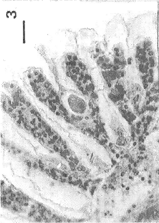
Fig.3: Microfotografía de una sección longitudinal de un foronte recién ingresado. H&E. Escala=25µm.
