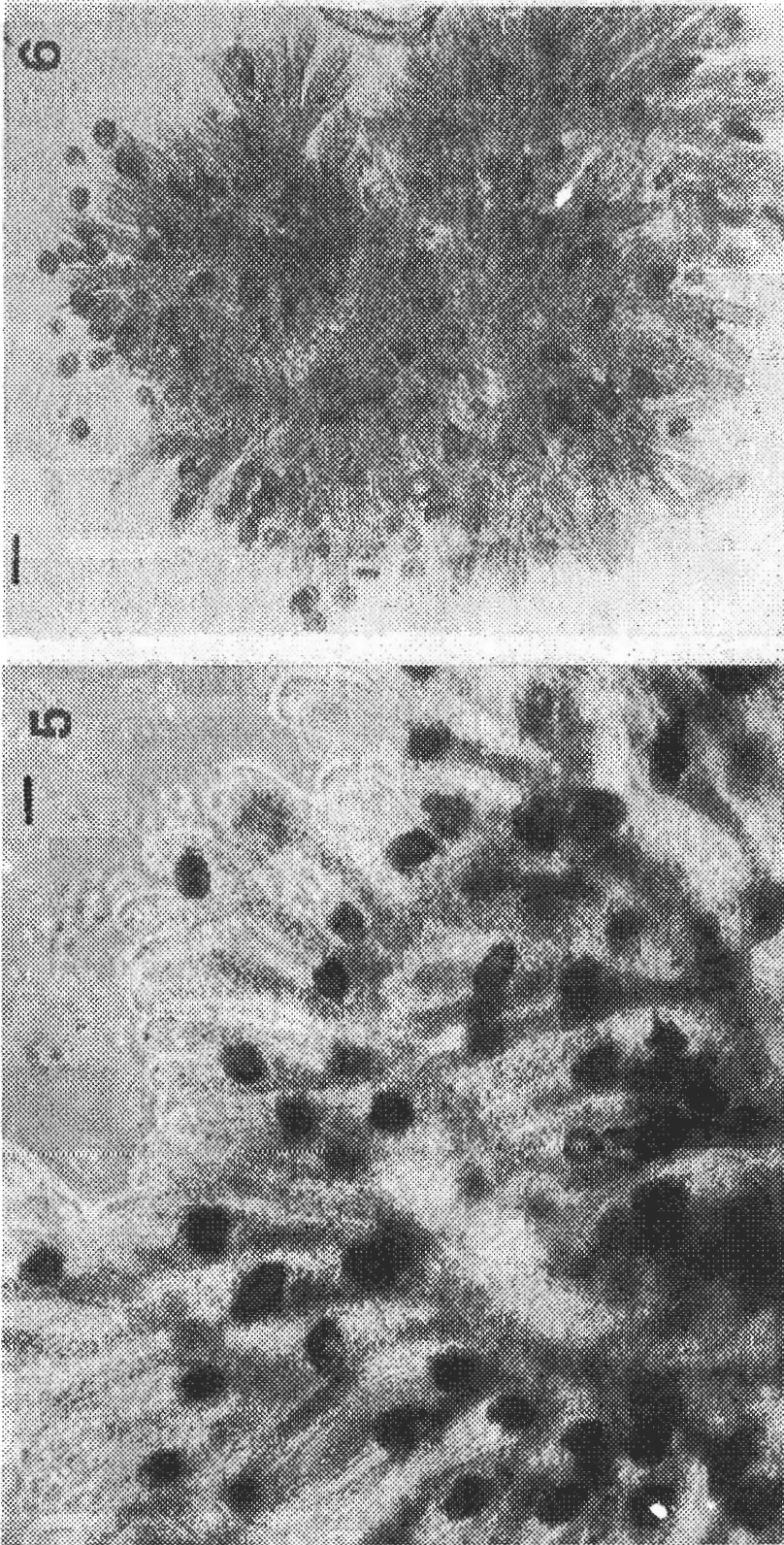
Fig.5: Microfotografía de branquias de A. longinaris con alta incidencia de A. longinaris con alta incidencia de A. longinaris con alta incidencia de A. longinaris con alta incidencia de A. longinaris . Escala=50 \mu m.
