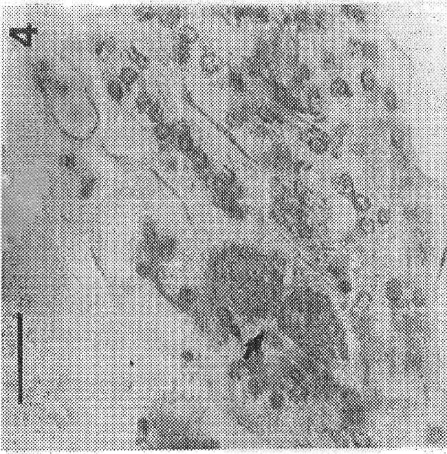
Fig.3: Microfotografía de una sección longitudinal de un foronte recién ingresado. H&E. Escala=25µm.
