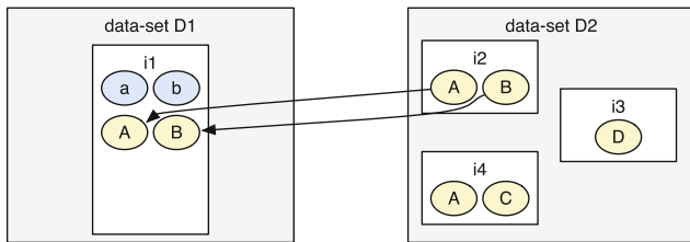
(b) instance enrichment ( topN=1 )
