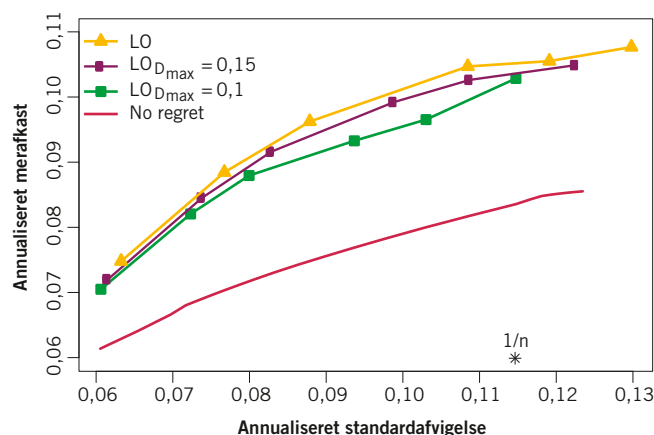
FIGUR 2: Den efficiente rand når risikoen måles som standardafvigelse.
