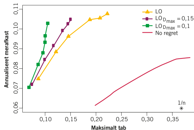
FIGUR 3: Den efficiente rand når risikoen måles som maksimalt tab.
