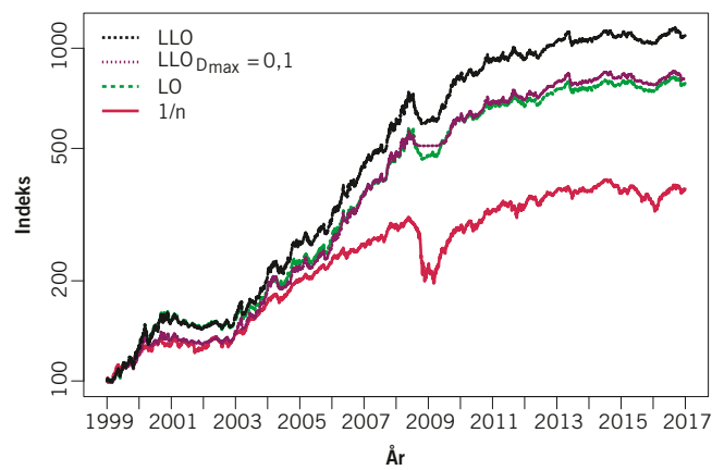
FIGUR 4: Afkastudviklingen for strategier med og uden gearing.
