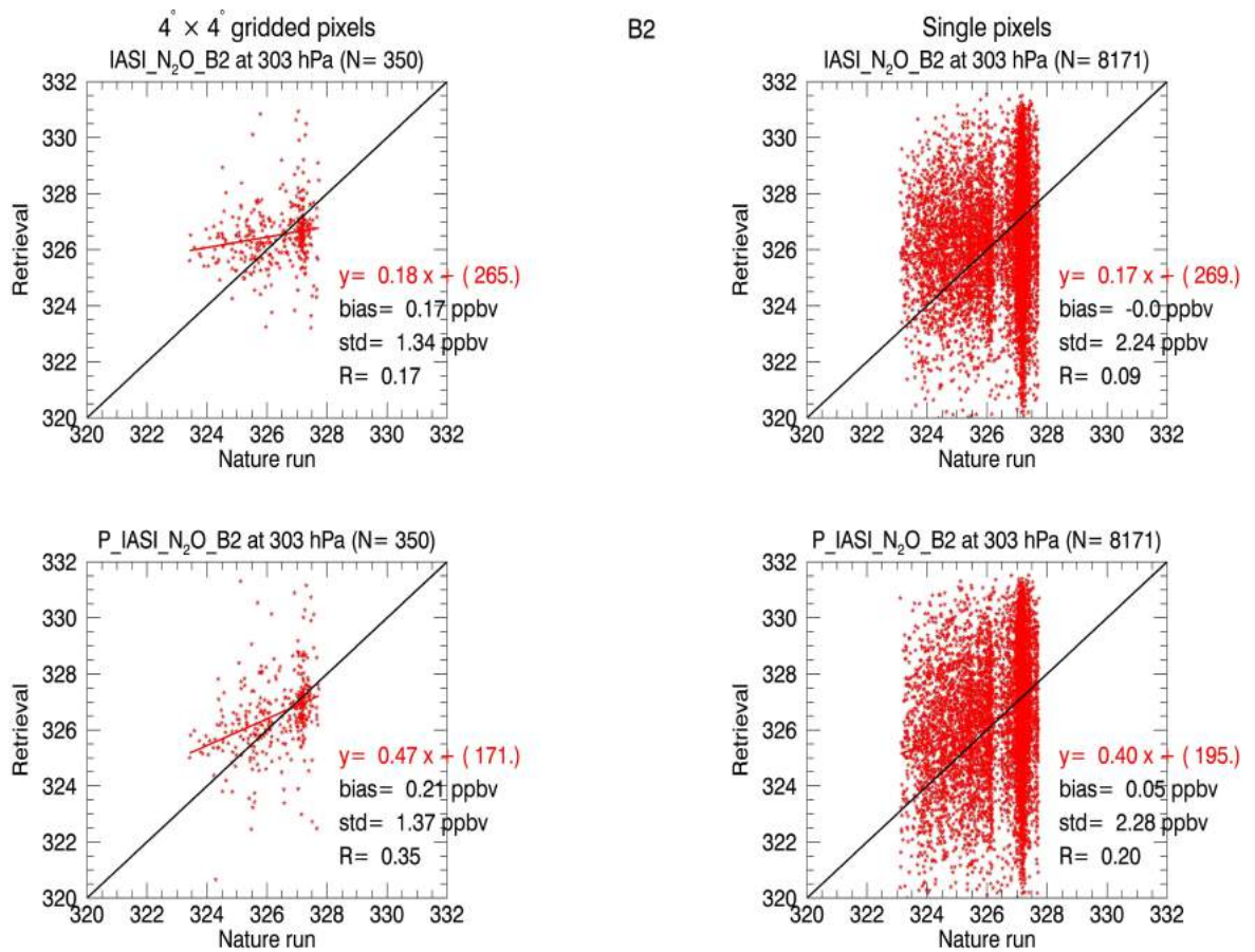
FIGURE B.9 – En haut (resp en bas) : nature-run vs IASI_N 2 O_B2 (resp P_IASI_N 2 O_B2) avec les pixels individuels (à droite) et moyennés sur une grille horizontale de 4° × 4° de résolution (à gauche). Sur chaque graphique, la droite rouge représente la droite de régression linéaire dont l'équation est écrite en rouge et la droite noire représente la première bissectrice.
