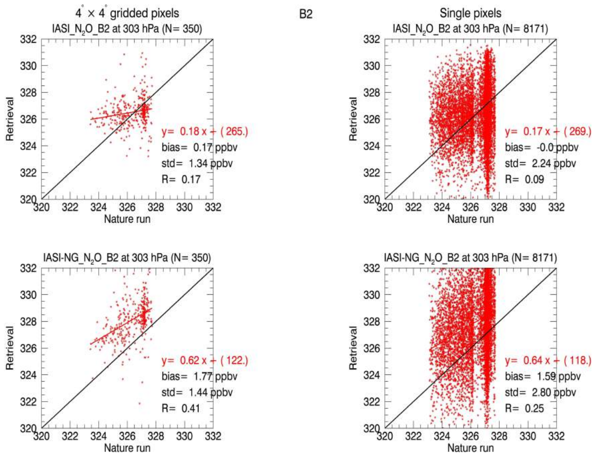
FIGURE 5.12 – En haut (resp en bas) : nature-run vs IASI_N 2 O_B2 (resp IASI-NG_N 2 O_B2) avec les pixels individuels (à droite) et moyennés sur une grille horizontale de 4° × 4° de résolution (à gauche). Sur chaque graphique, la droite rouge représente la droite de régression linéaire dont l'équation est écrite en rouge et la droite noire représente la première bissectrice.
