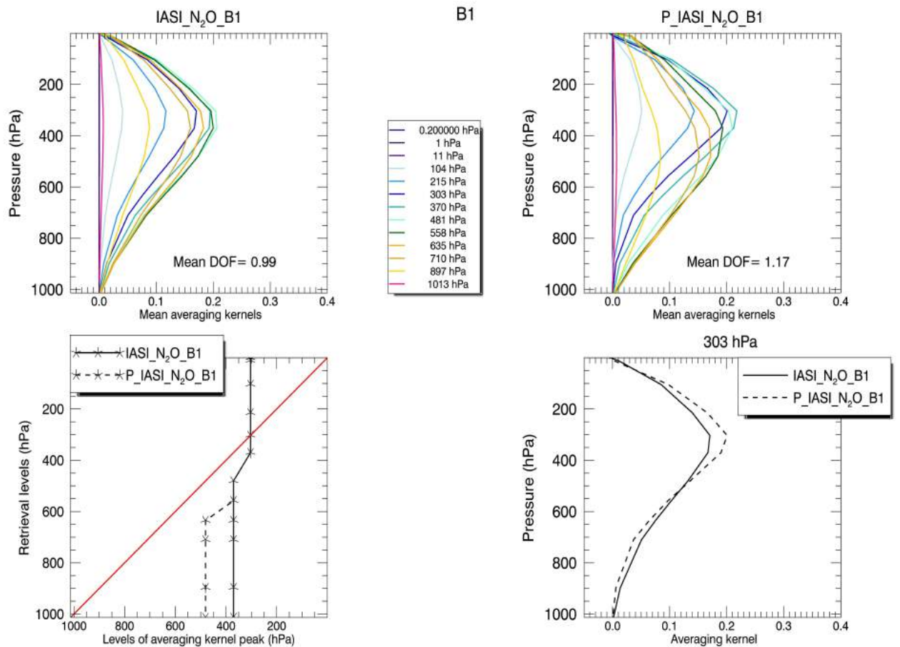
FIGURE B.2 – Fonctions de balayage (en haut) de N 2 O moyennées sur l’orbite de référence pour IASI_N 2 O_B1 (à gauche) et P_IASI_N 2 O_B1 (à droite). Altitudes des maxima des fonctions de balayage moyens (en bas à gauche) et fonctions de balayage moyens du niveau 303 hPa (en bas à droite) pour IASI_N 2 O_B1 (traits pleins) et P_IASI_N 2 O_B1 (tirets).
