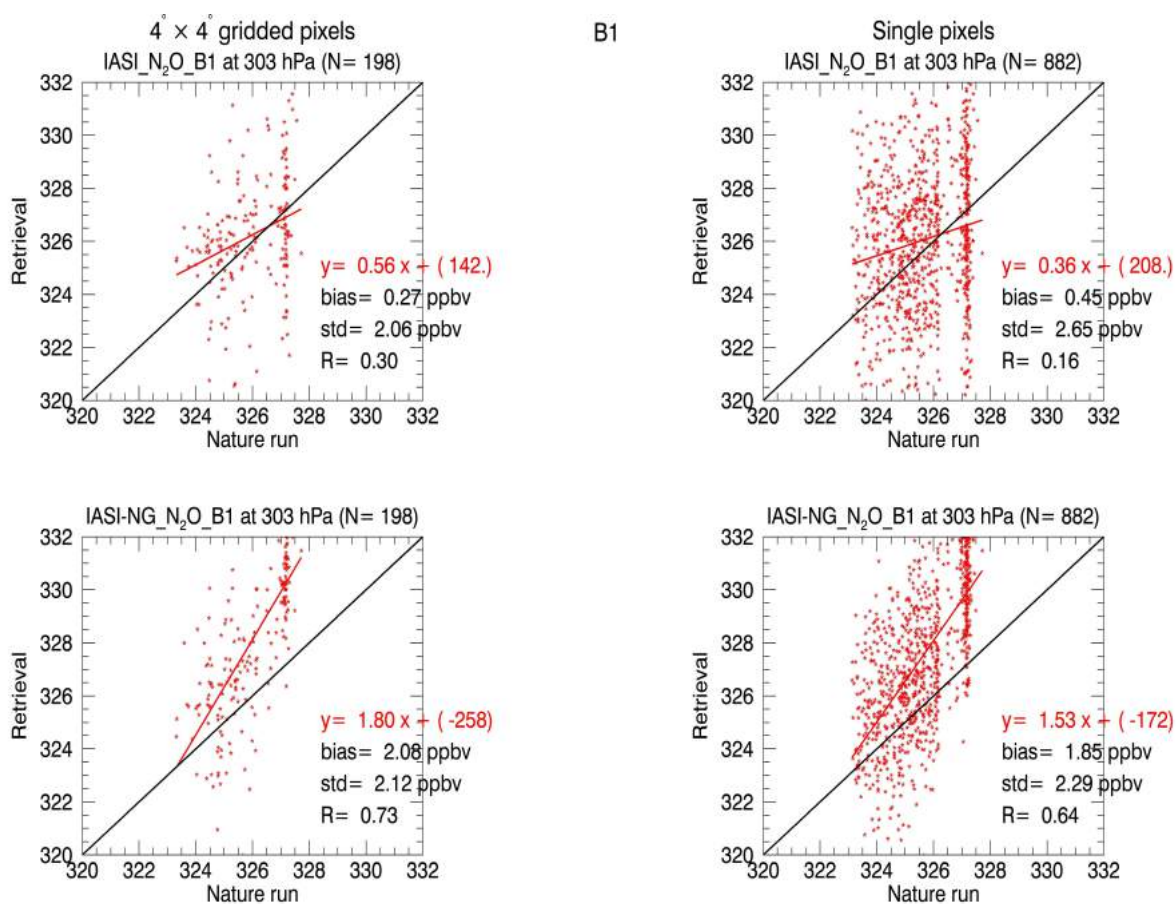
FIGURE 5.11 – En haut (resp en bas) : nature-run vs IASI_N 2 O_B1 (resp IASI-NG_N 2 O_B1) avec les pixels individuels (à droite) et moyennés sur une grille horizontale de 4° × 4° de résolution (à gauche). Sur chaque graphique, la droite rouge représente la droite de régression linéaire dont l'équation est écrite en rouge et la droite noire représente la première bissectrice.
