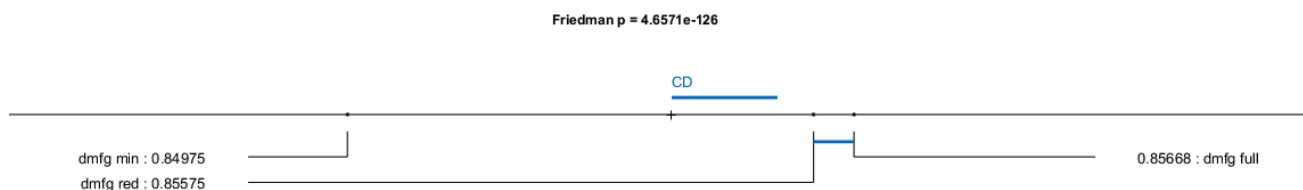
FIGURE 4.26 – Résultats du test de Friedman avec post-hoc de Nemenyi entre les échantillons représentant les différents ensembles de méta-attributs généraux utilisés.
