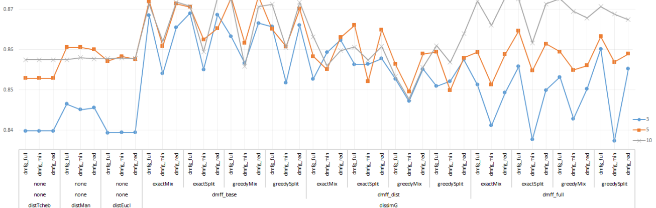
FIGURE 4.12 – Moyenne des performances au méta-niveau selon le nombre k de voisins considérés.
