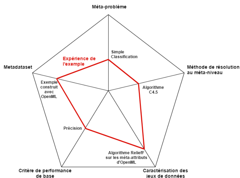
FIGURE 3.1 – Dimensions considérées dans l'exemple
