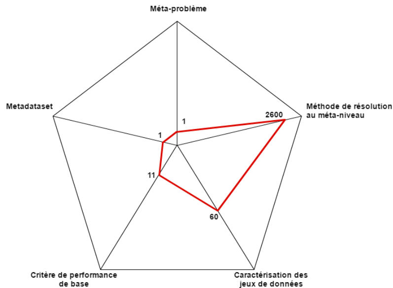
FIGURE 3.2 – Taille des dimensions d'expérimentation
