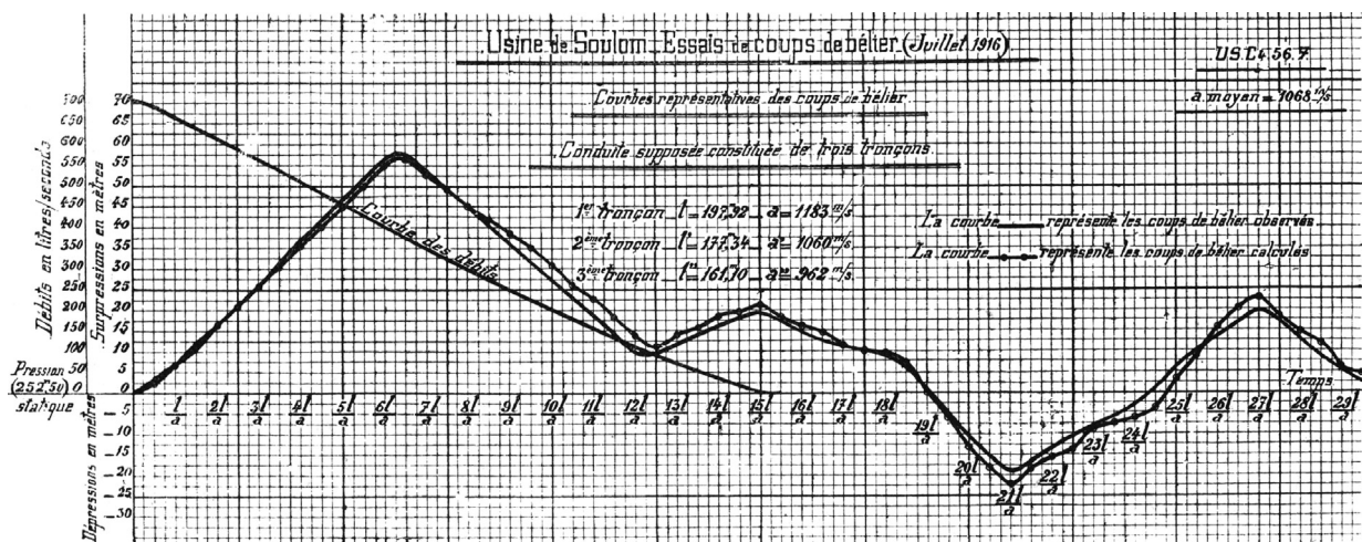
Fig. 10. Fermeture lente du distributeur au pied de la conduite forcée de l'usine de Souloin : pression au distributeur en fonction du temps, mesure et calcul pour une conduite représentée par trois tronçons d'épaisseurs différentes [5].
