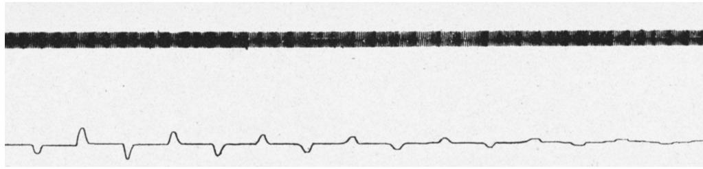
Fig. 9. Enregistrement de la pression après une brève ouverture d'un petit robinet à l'aval d'une conduite (méthode de la dépression brusque); au-dessus : enregistrement d'un diapason au 1/100s donnant l'échelle de temps [5].
