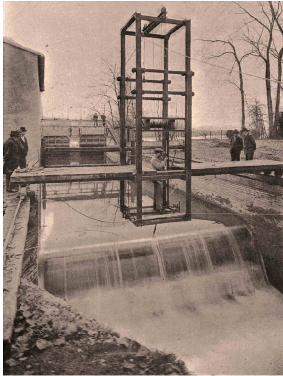
Fig. 3. Le canal courbe du laboratoire de Baniève, et nacelle de mesure du débit à l'aide du déversoir de Bazin (Arch. IMFT).
