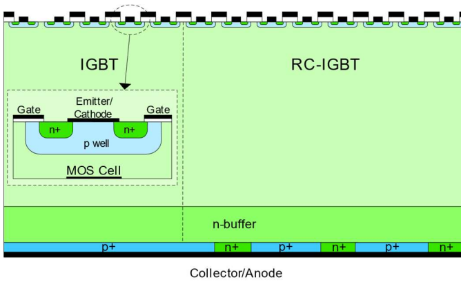
Fig. 13. BIGT structure [16].
