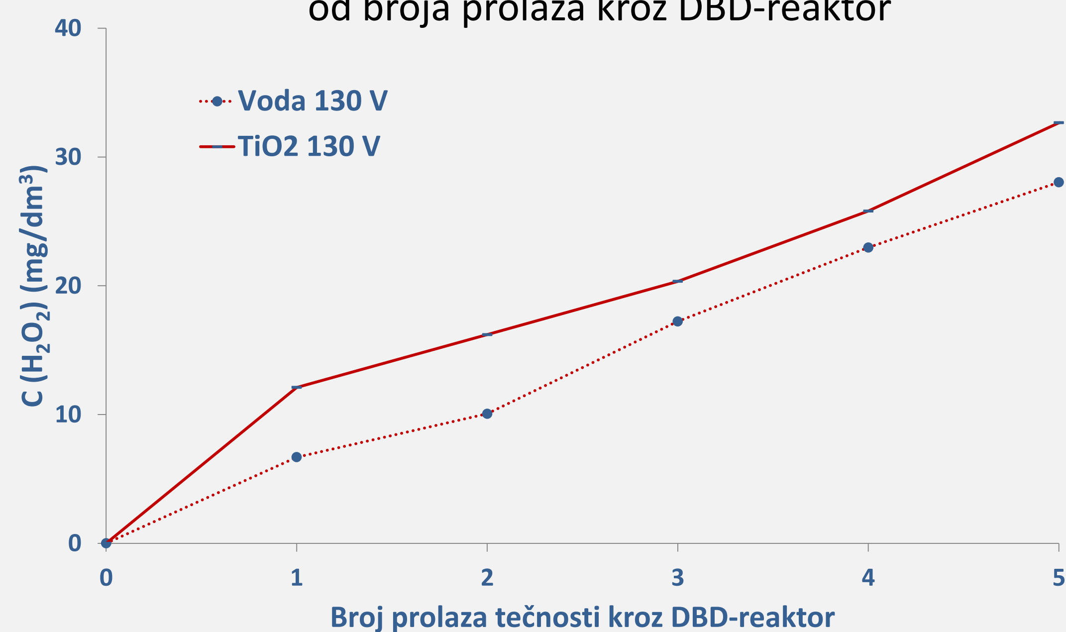
Grafik 1. Zavisnost C(\text{H}_2\text{O}_2) u vodi i u suspenziji \text{TiO}_2 od broja prolaza kroz DBD-reaktor
