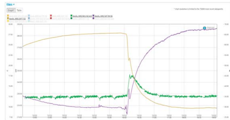
Figura 7. Efecto de una variación brusca de humedad relativa (lila) sobre la señal del sensor de NO 2 (verde).
