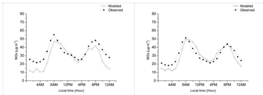
Figura 5. Comparación entre las concentraciones horarias de NOx modeladas y observadas. Día promedio anual en: a) Pamplona-Iturrama, b) Pamplona-Rotxapea.
