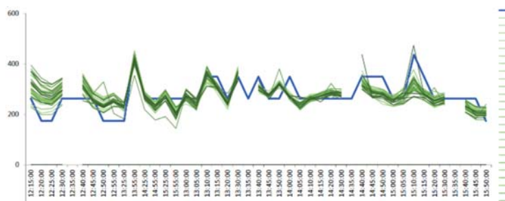
Figura 8. Lecturas de sensores co-localizados para un mismo contaminante antes y después de la fase final de correcciones de intercalibración.
