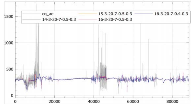
Figura 6. Señal original de uno de los electrodos del sensor de CO, en gris, y procesada con diversos ajustes de los filtros de detección de interferencias.
