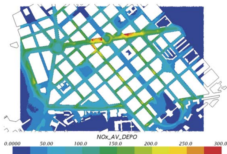
Figura 3. Mapa de alta resolución de concentración de NOx ( \mu\text{g}/\text{m}^3 ) promedio durante el periodo del 1 al 14 de marzo de 2015 estimado por el modelo CFD para el distrito de Plaza de la Cruz (Pamplona).
