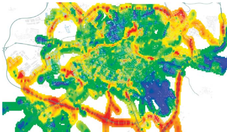
Figura 10. Niveles medios de \text{NO}_2 en una escala del azul (bajo) al rojo (alto) entre las 8h y las 9h de la mañana. Los mayores niveles corresponden a las vías de más tráfico y circulación más rápida, como circunvalaciones o ejes de varios carriles. Hay puntos de alta concentración en cruces y algunos colegios. El color rojo corresponde a niveles por encima de 40 ppb, indicador de una calidad del aire deficiente.
