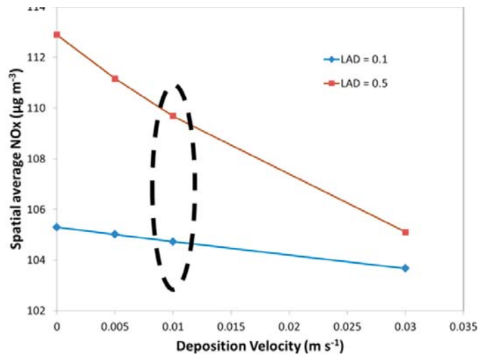
Figura 6. Variación de la concentración espacial media de NOx a 3 m sobre el suelo en función de las velocidades de depósito de contaminantes por la vegetación para dos densidades de follaje (LAD).
