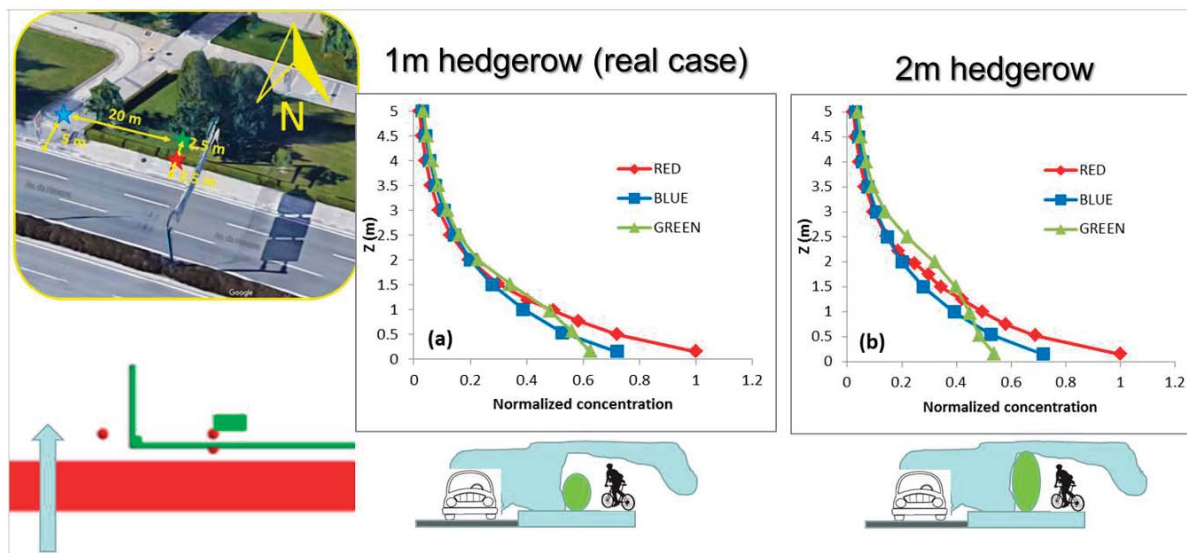
Figura 8. Resultados de las simulaciones de los experimentos del efecto de setos en la calidad del aire para el caso real de seto de 1 m de altura y otro hipotético de 2 m. Los colores de las curvas se corresponden con los puntos de medida en las campañas de campo, tal como se muestra en la imagen superior izquierda.
