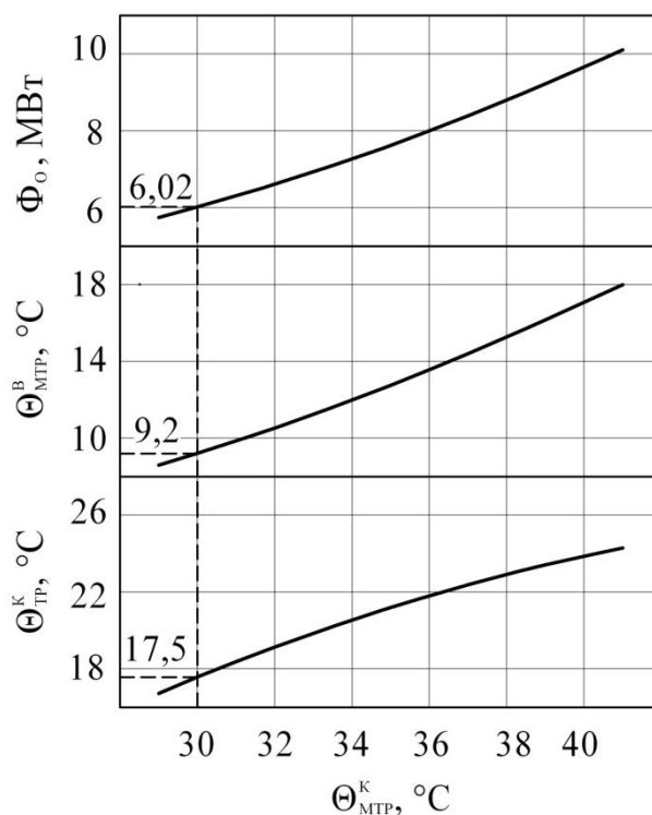
Рис. 1 Вплив температури ЦГ на вході конденсаційної колони \Theta_{MTP}^K на розподіл температур на вході випарників \Theta_{MTP}^B , на виході трубного простору конденсаційної колони \Theta_{TP}^K та холодопродуктивність \Phi_0 випарників за постійної температури охолодження \Theta_{TP}^B = -5^{\circ}\text{C}
