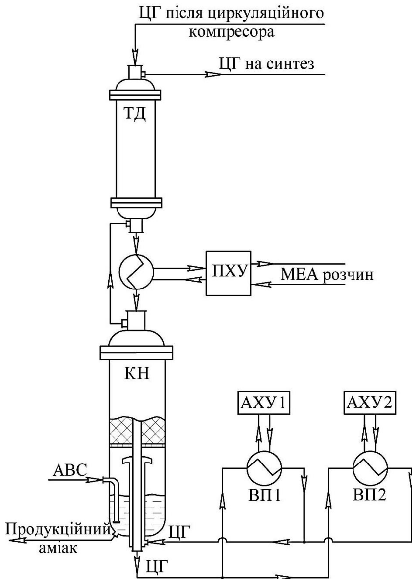
Рис. 3 Апаратурно-технологічне оформлення комплексу вторинної конденсації підвищеної енергоефективності: КН – конденсаційна колона; ЦГ – циркуляційний газ; АВС – азотно-воднева суміш; АХУ – абсорбційно-холодильна установка; ПХУ – пароежекторна холодильна установка; ВП – випарник; ТД – додатковий теплообмінник
