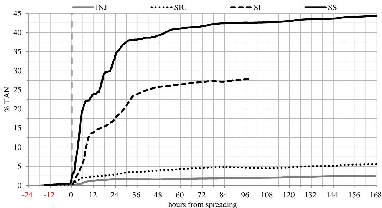
Fig.1 – Flussi cumulate di ammoniac ( \text{NH}_3 ) come percentuale di azoto ammoniacale applicato (%TAN), ottenuti usando il modello WindTrax (si veda testo per riferimenti sul modello) per differenti tecniche di spandimento: iniezione (INJ), spandimento superficiale senza incorporazione (SS), incorporazione superficiale a 24 ore (SI), e contemporaneamente allo spandimento (SIC).
