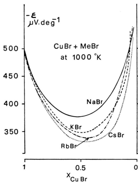
Fig. 2. \varepsilon_{750} \text{ } ^\circ\text{C} vs x_{\text{CuBr}} .
