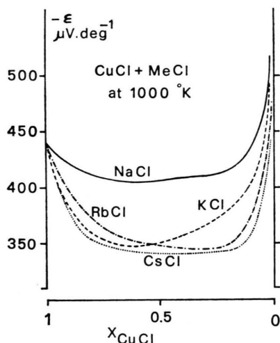
Fig. 1. \varepsilon_{801} \text{ } ^\circ\text{C} vs x_{\text{CuCl}} .
