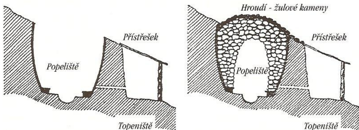
Obrázek 2: Výtavba milíře [7]
