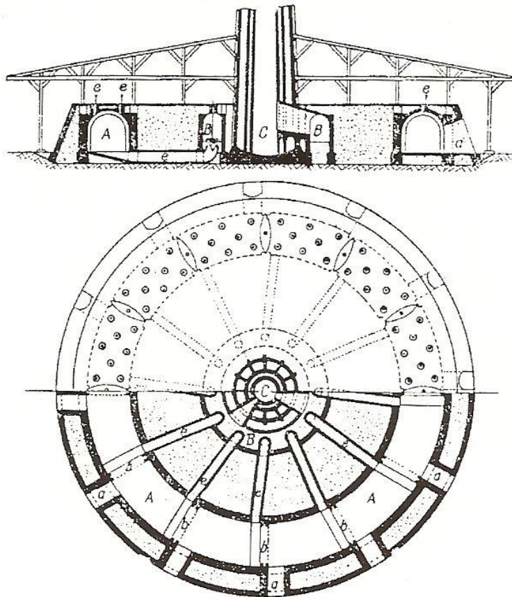
Obrázek 3: Hoffmannova kruhovka [25]
