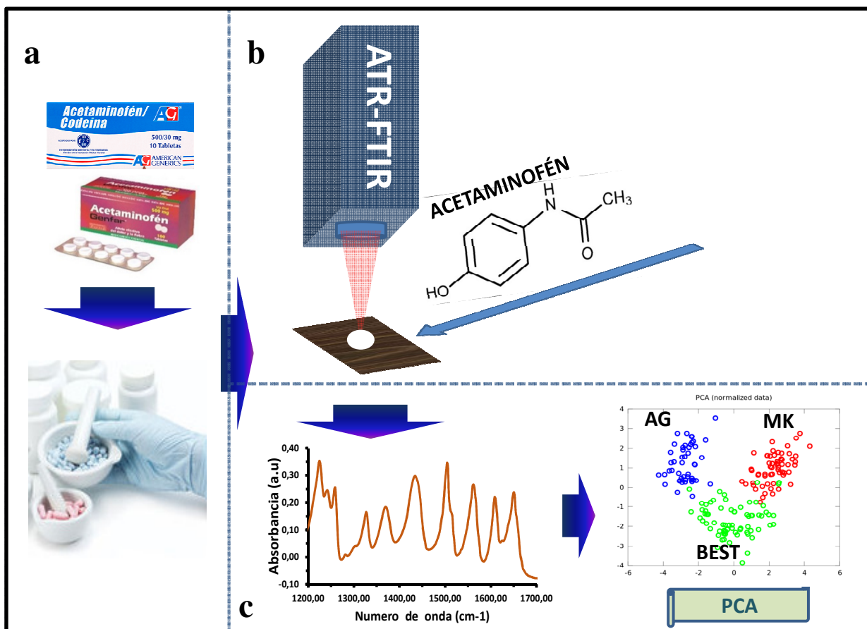
Fig. 1 Configuración Experimental para la detección de AAP sólido presente en diferentes productos farmacéuticos.
