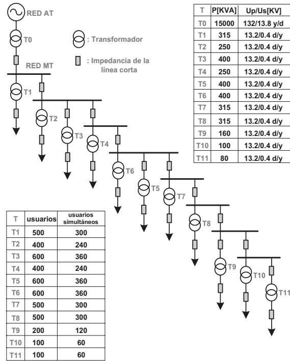
Fig. 11. Diagrama unifilar reducido de la red analizada. Fuente: Autores.
