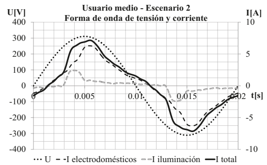
Fig. 10b. Forma de onda de tensión y corriente de un usuario medio correspondiente al escenario 2 Fuente: Autores.
