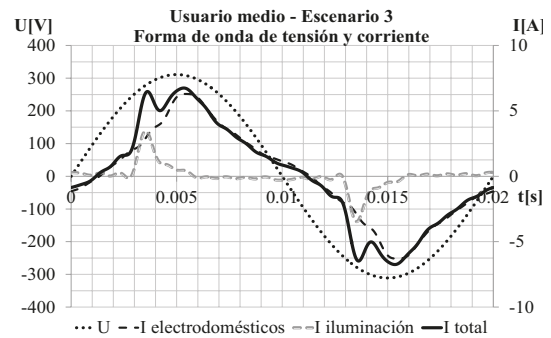
Fig. 10c. Forma de onda de tensión y corriente de un usuario medio correspondiente al escenario 3 Fuente: Autores.
