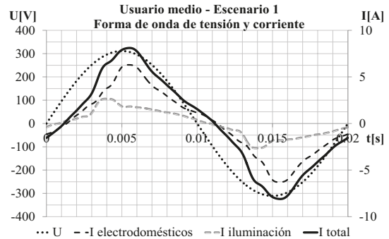
Fig. 10a. Forma de onda de tensión y corriente de un usuario medio correspondiente al escenario 1 Fuente: Autores.
