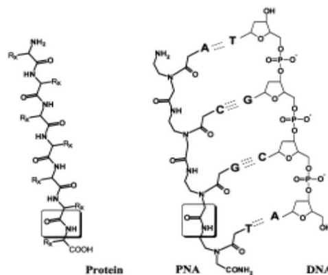
Figura 6: Comparação estrutural entre a proteína e o PNA interagindo com uma fita de DNA.
